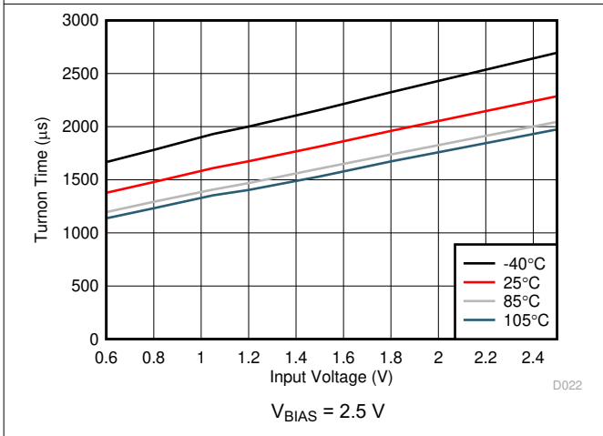
图 6-27. Turnon Time vs Input Voltage
