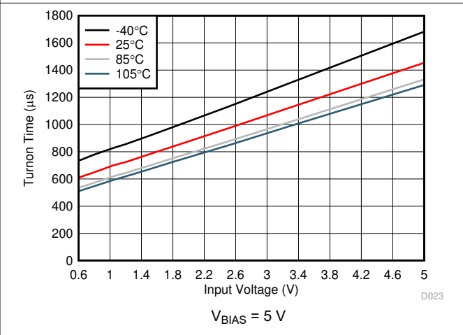
图 6-28. Turnon Time vs Input Voltage
