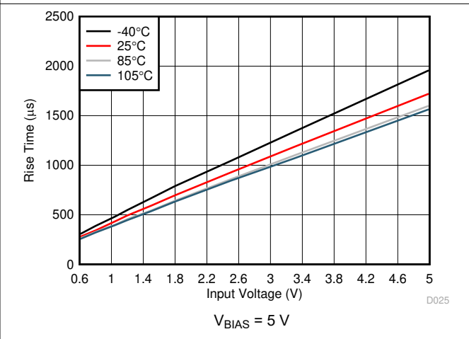
图 6-30. Rise Time vs Input Voltage
