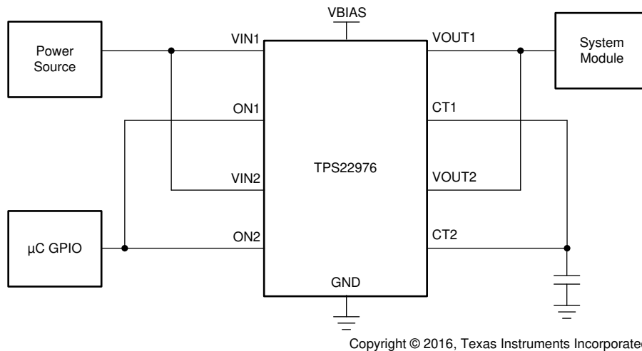
图 9-1. Parallel Configuration
