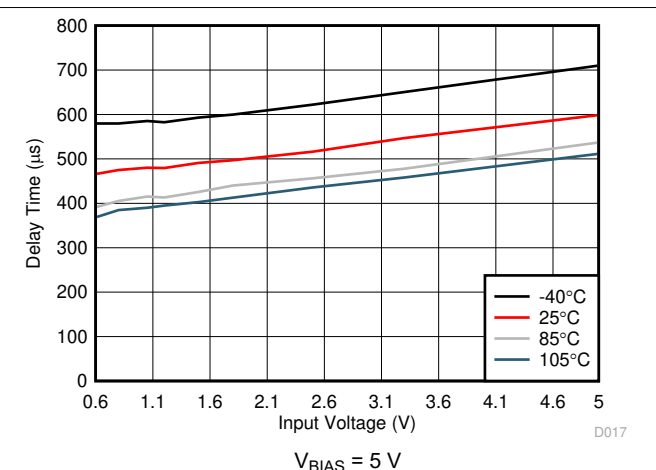
图 6-20. Delay Time vs Input Voltage
