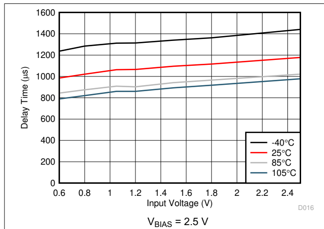
图 6-19. Delay Time vs Input Voltage
