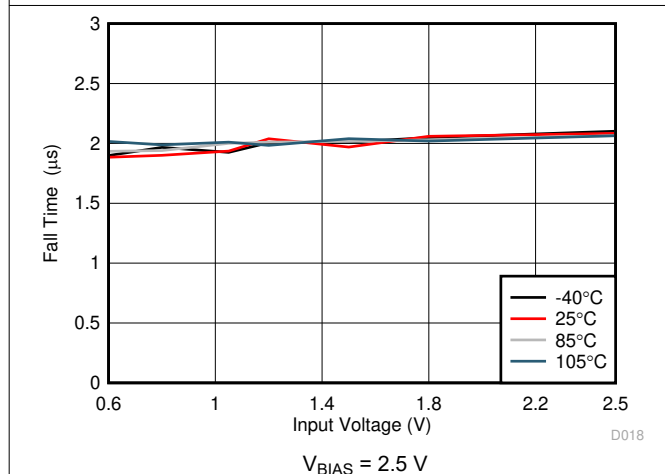
图 6-21. Fall Time vs Input Voltage
