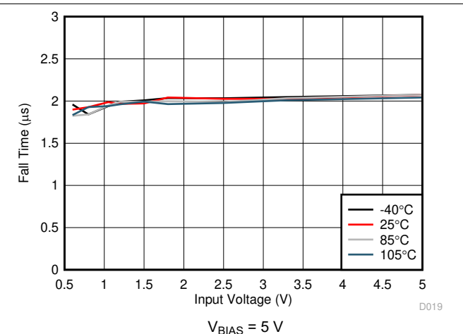
图 6-22. Fall Time vs Input Voltage
