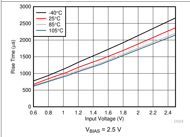
图 6-29. Rise Time vs Input Voltage
