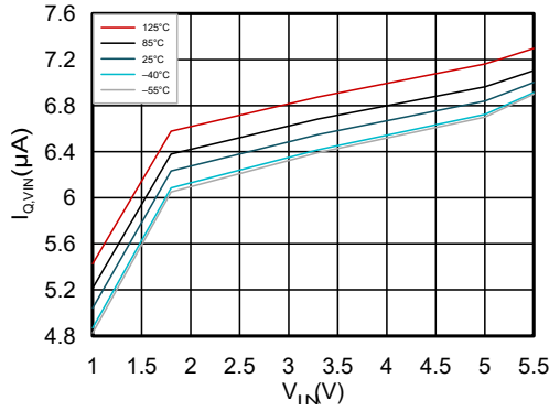
图 6-1. V IN 静态电流与输入电压间的关系
