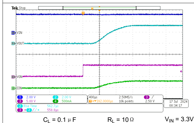
图 9-4. TPS22991C 的典型导通
