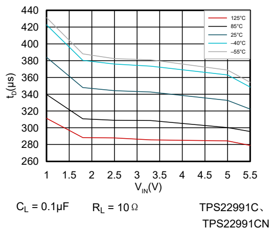
图 6-13. 延迟时间与输入电压间的关系
