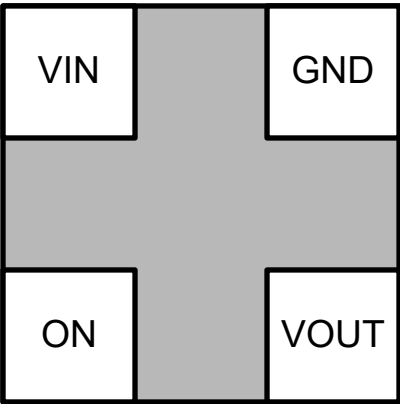
图 5-1. TPS22991 RAA 封装，4 引脚 UQFN ( 顶视图 )
