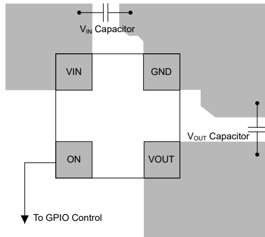
图 9-6. TPS22991I 布局
