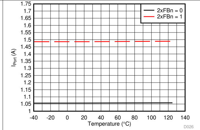
图 26. I_SHORT 阈值与温度间的关系
