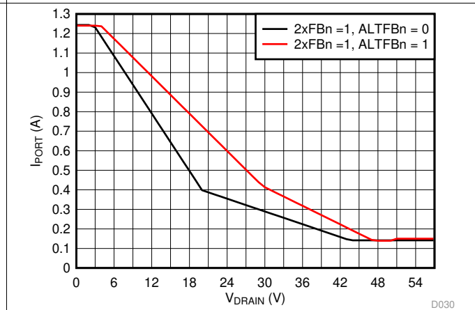
图 30. 2x 模式 (2xFBn = 1) 电流折返与漏极电压间的关系
