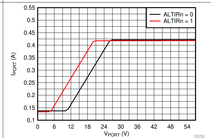
图 28. 浪涌电流折返与端口电压间的关系
