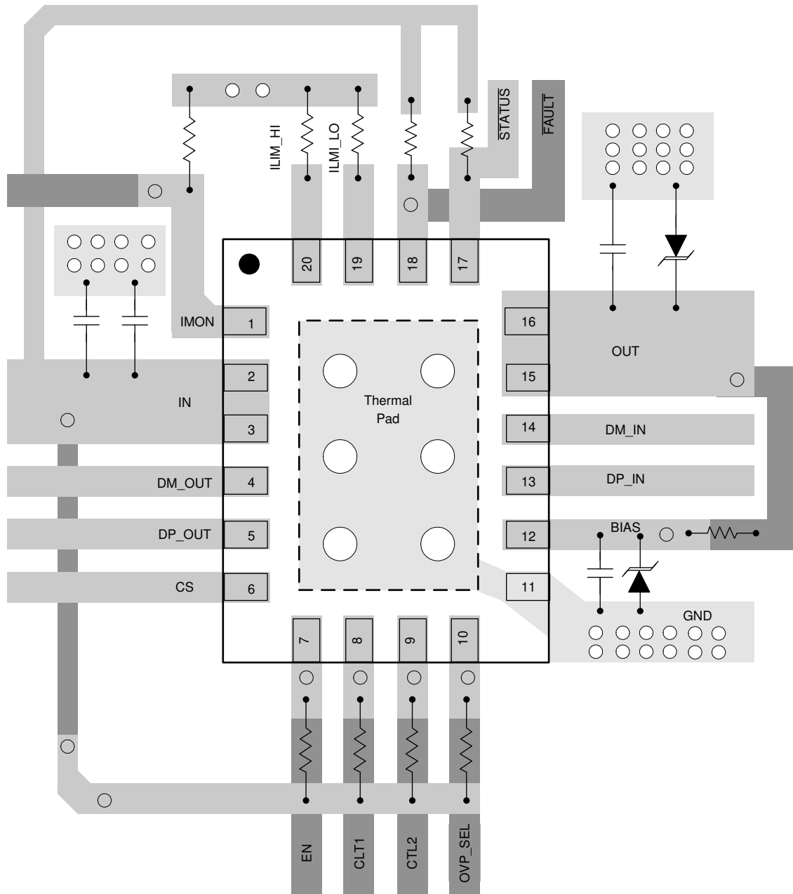
图 11-1. TPS254900A-Q1 Layout Diagram
