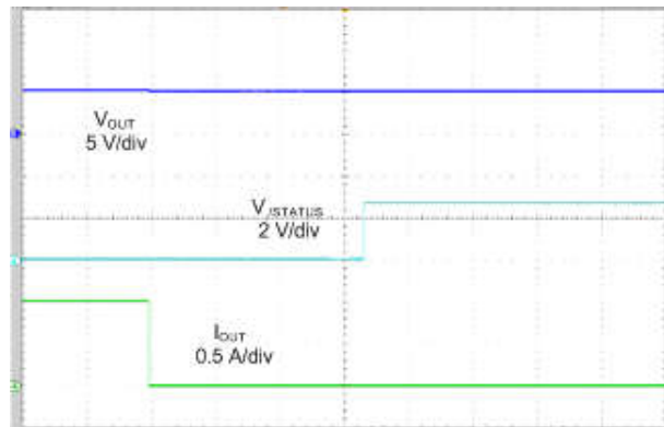
图 6-24. Hot Short
