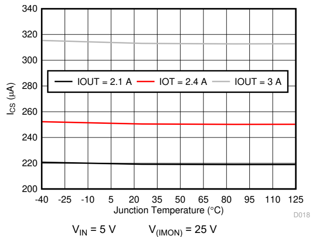
图 6-14. I (IMON) vs Temperature
