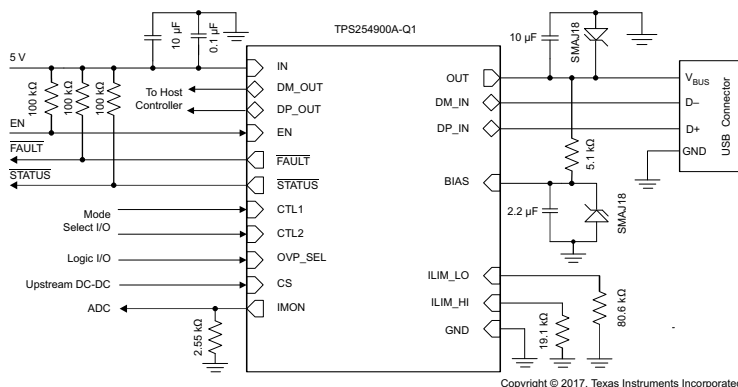
原理图
