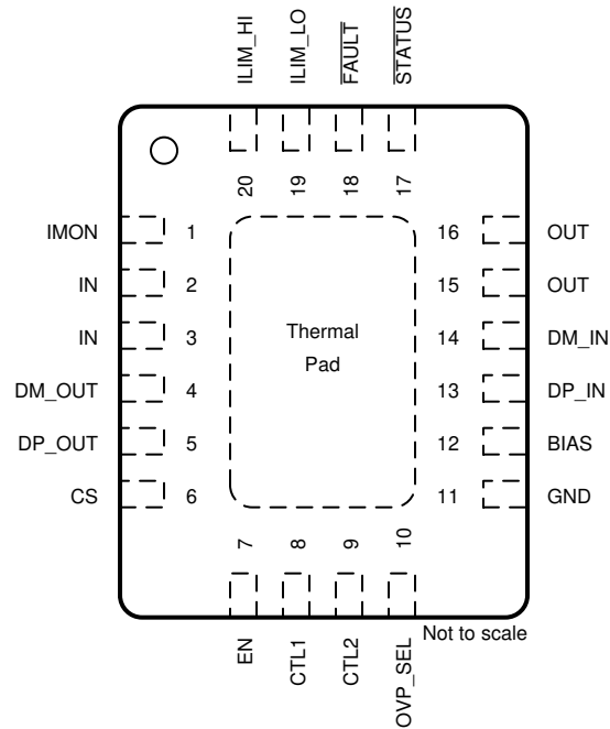
图 5-1. RVC Package 20-Pin WQFN Top View
