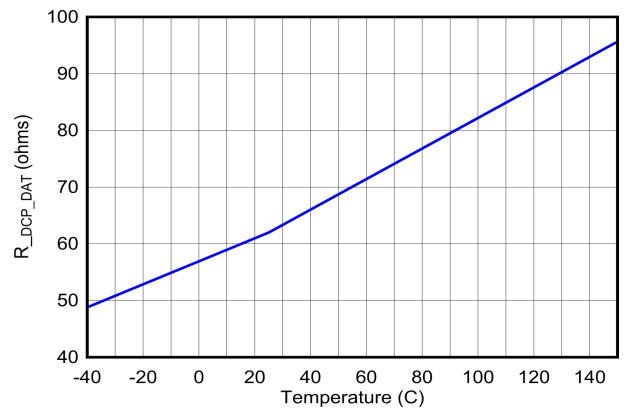
图 6-42. USB BC1.2: DP 至 DM 短路电阻 R_{DCP\_DAT} 与温度间的关系
