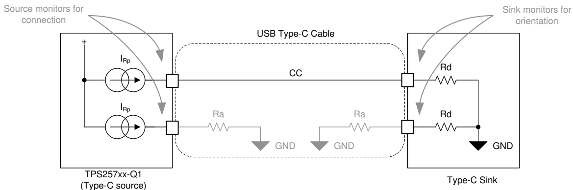
图 8-28. Type-C 电缆
