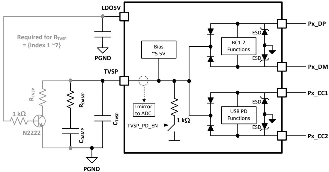
图 8-5. R_{TVSP} 电路配置
