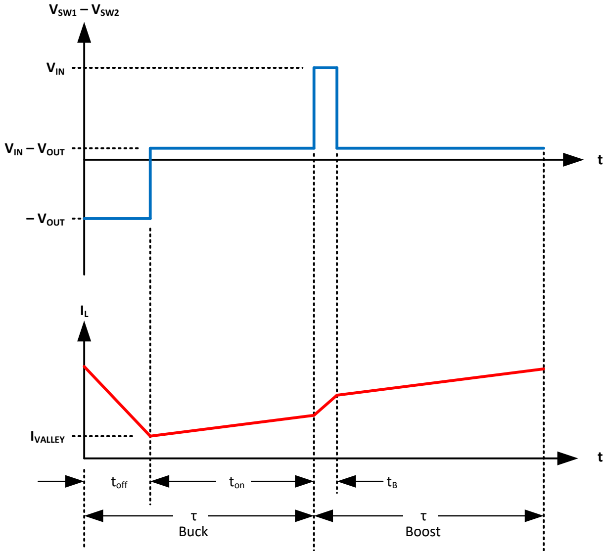
图 8-9. 降压转换
