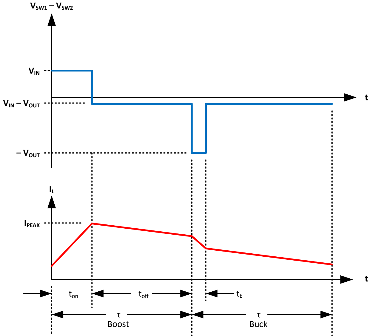
图 8-10. 升压转换
