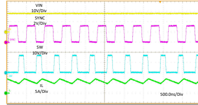
VIN = 18 V L = 0.68 uH I PA_BUS = 3 A I PB_BUS = 3 A
