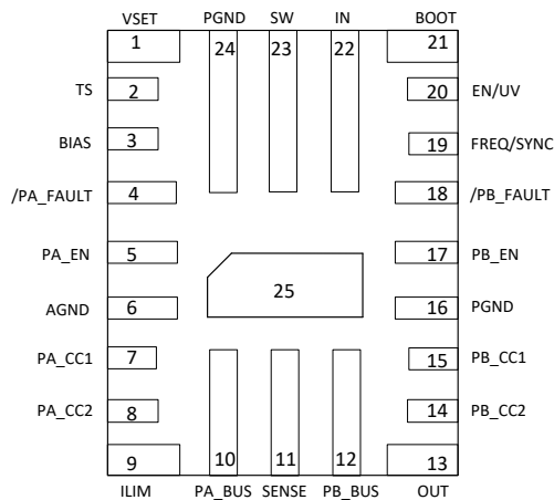
图 7-3. TPS25852-Q1 RPQ Package 25-Pin (QFN) Top View
