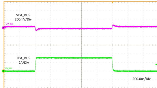
图 11-5. Load Regulation
