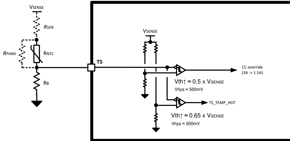
图 10-16. TS Input
