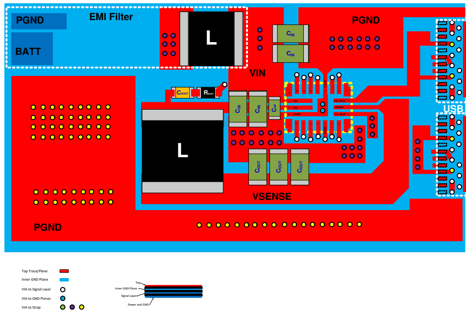
图 13-1. Layout Example
