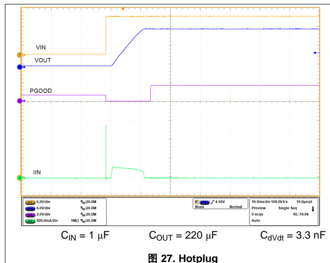
图 27. Hotplug
