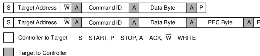
图 8-12. Write Byte
