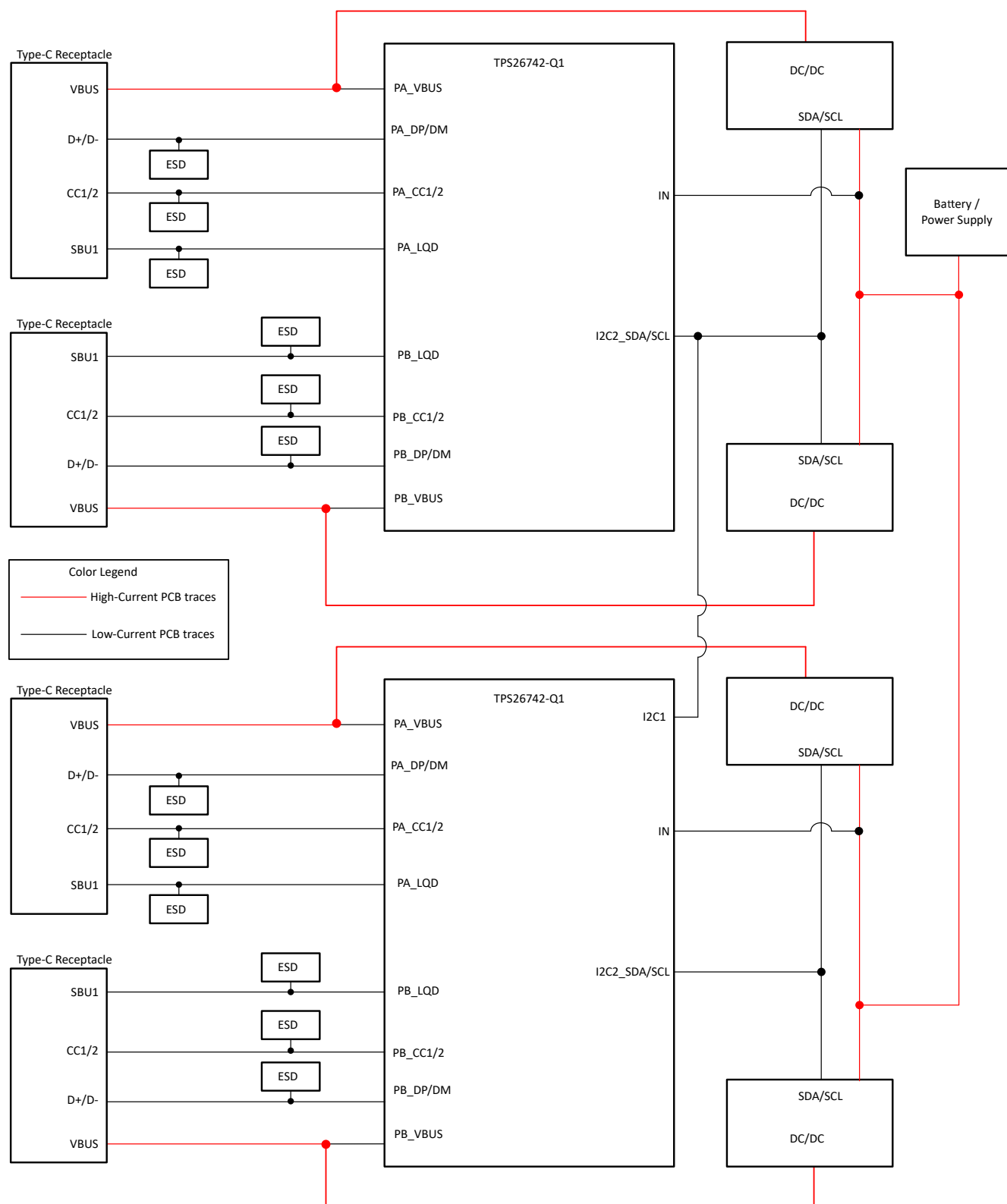
图 9-2. 双端口 SPR 充电器
