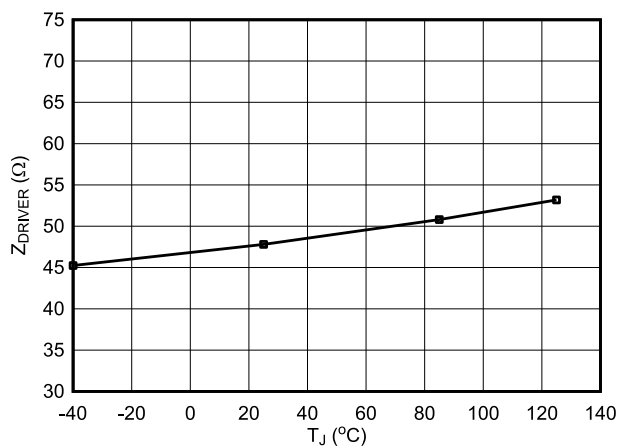
图 6-2. USB-PD PHY 发送阻抗
