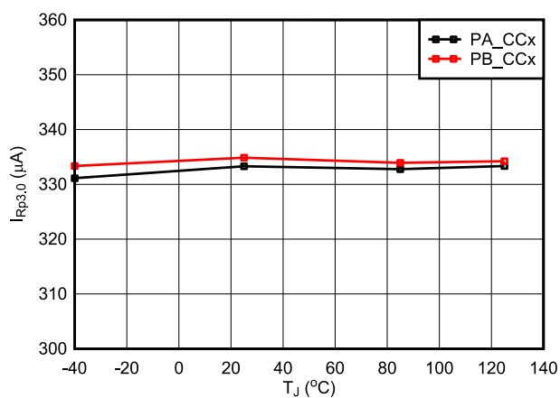
图 6-6. 广播 3A 电缆检测电流源的强度
