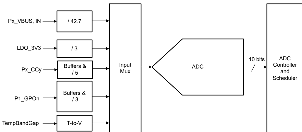
图 8-22. SAR ADC
