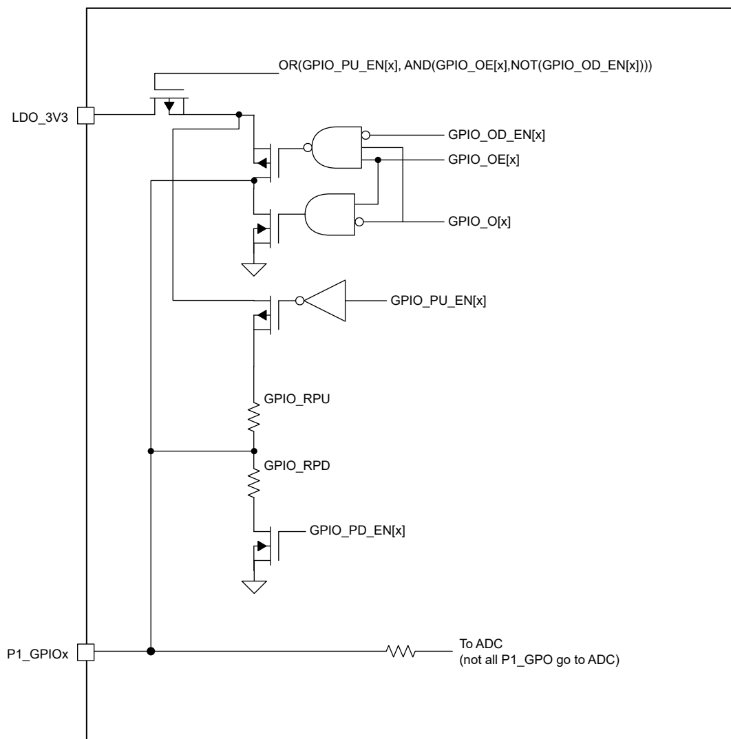
图 8-26. P1_GPOx 缓冲器
