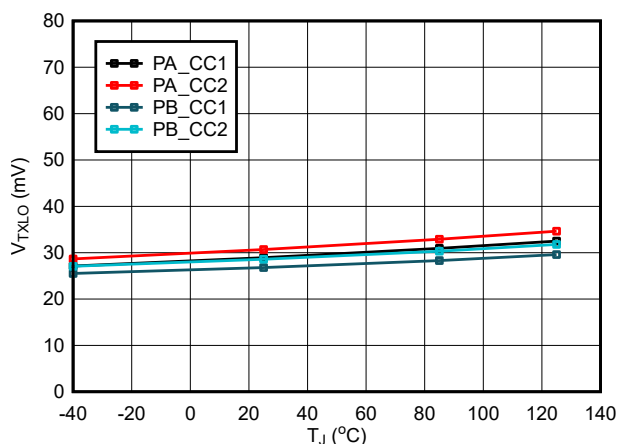
图 6-4. USB-PD PHY 发送低电压
