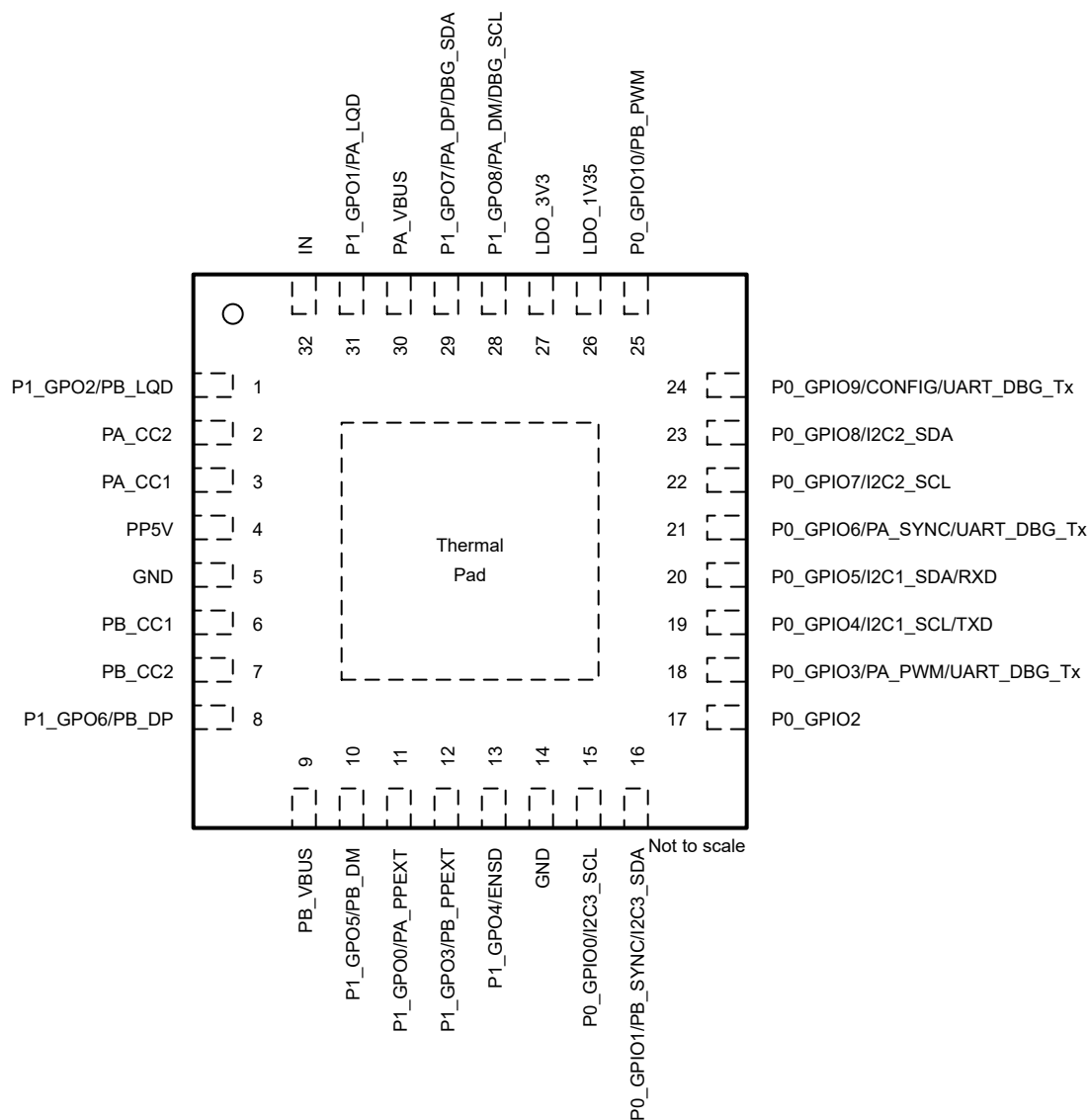
图 5-1. TPS26742-Q1 RHB 封装, 32 引脚 QFN (顶视图)
