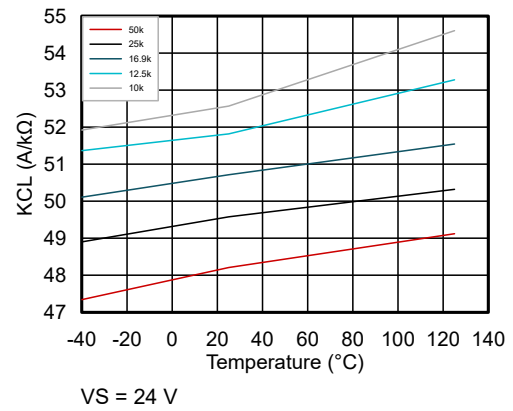
图 6-10. 电流限制比 ( K_{CL} ) 与温度与 R_{ILIM} 间的关系
