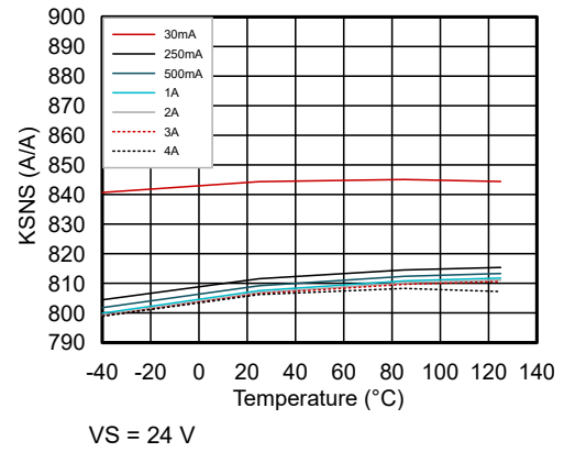
图 6-8. 电流检测比 ( KSNS ) 与温度和负载电流间的关系
