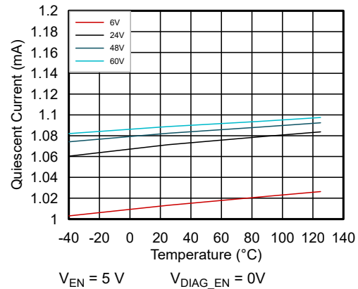
图 6-2. 来自 VS 输入电源的静态电流 ( I_{Q,vs} ) 与温度与 VS 电压间的关系 V_{EN} = 5\text{ V} V_{DIAG\_EN} = 0\text{ V}
