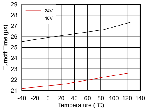
图 6-7. 关断时间 ( t_{OFF} ) 与温度与 V_S 电压间的关系
