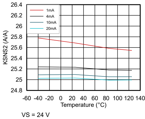
图 6-9. 电流检测比 ( KSNS_2 ) 与温度与负载电流间的关系
