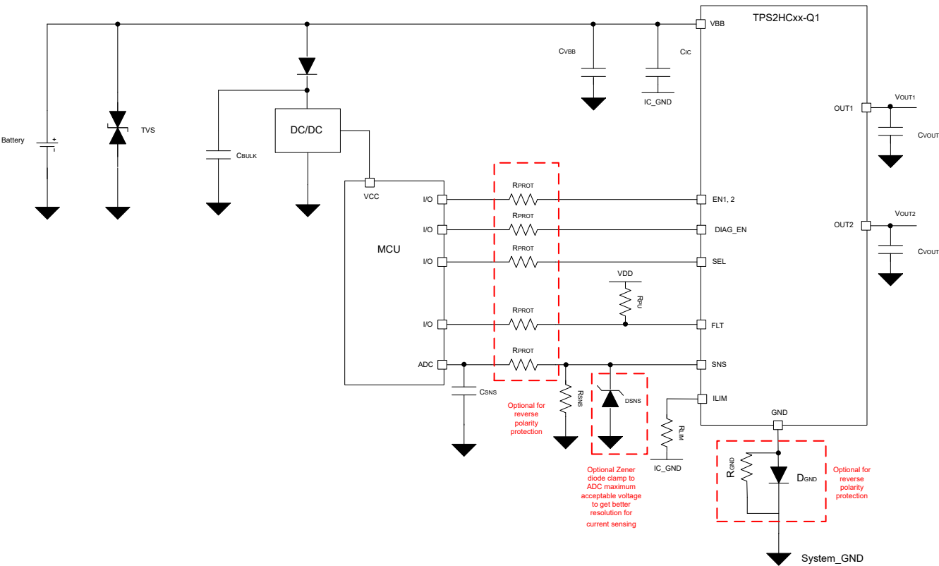
图 9-1. 典型应用图
