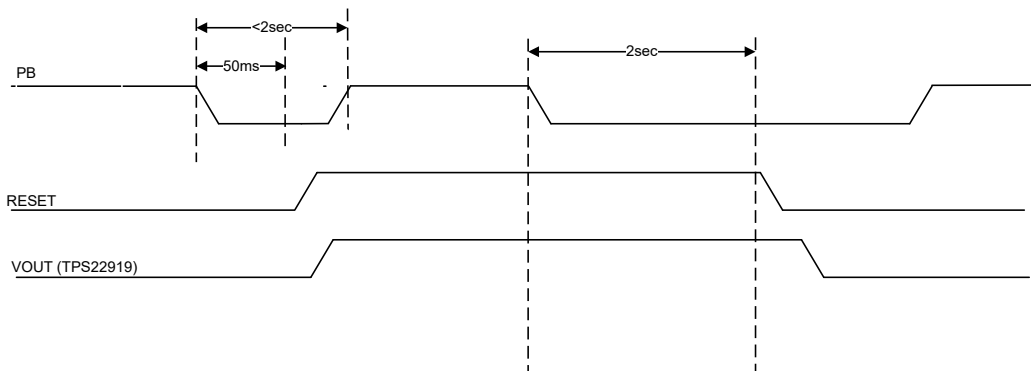
图 8-2. 通过负载开关进行功率控制
