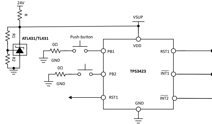
图 8-3. 通过 ATL431 提供高压支持
