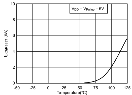
图 6-11. 开漏 RESET 漏电流与温度间的关系
