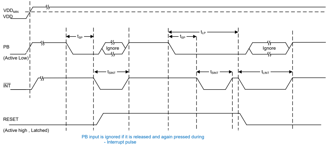
图 6-1. 时序图：锁存 RESET
