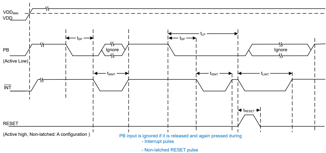
图 6-3. 时序图：非锁存 RESET
