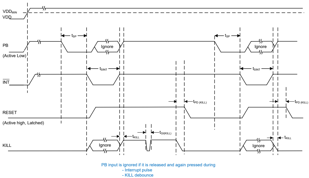
图 6-5. 时序图 : KILL
