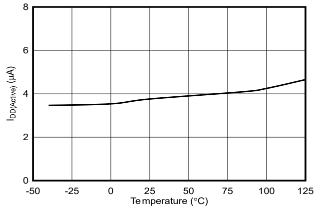
图 6-7. 有效电流与温度间的关系 (低电平有效按钮输入)
