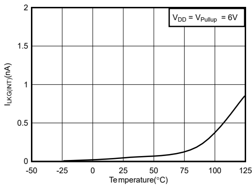
图 6-10. INT 漏电流与温度间的关系
