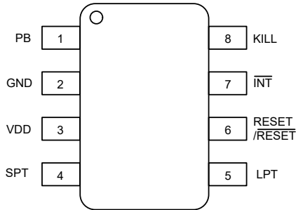
图 5-3. 引脚配置选项 TPS3424 DRL 封装 8 引脚 SOT-23 顶视图
