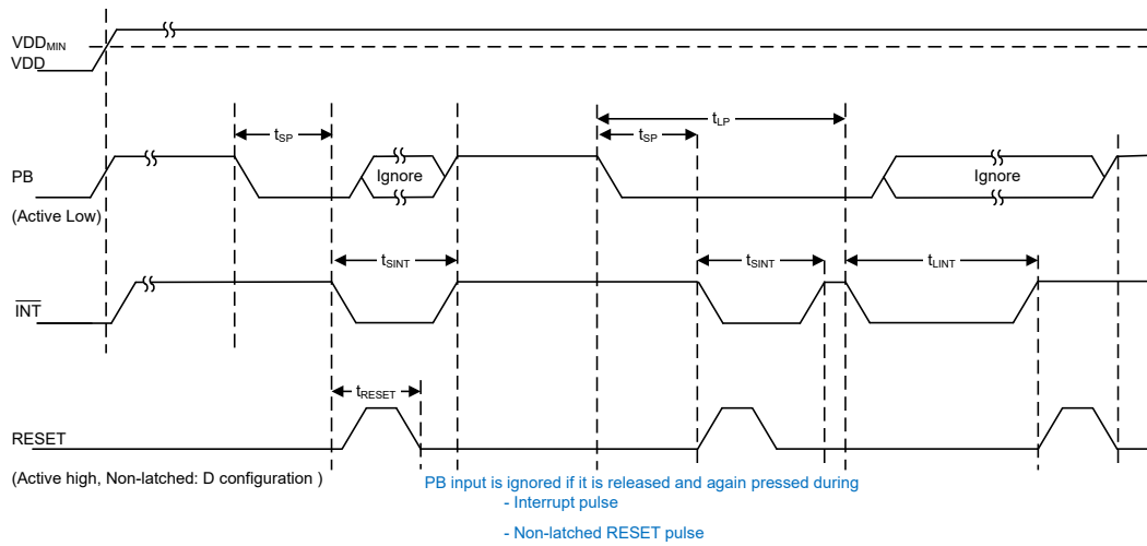
图 6-4. 时序图 : 非锁存 RESET ( SP : INT 时复位 , LP : INT 后复位 )
