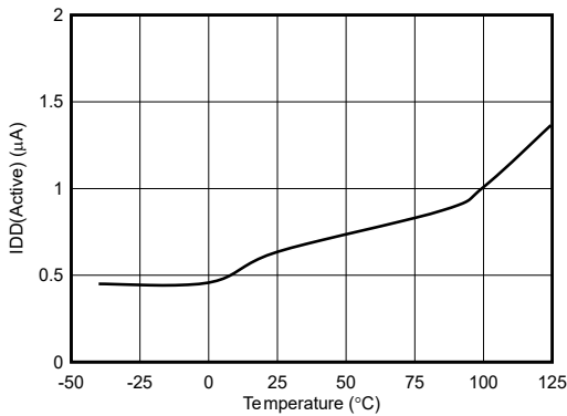
图 6-8. 有效电流与温度间的关系 (高电平有效按钮输入)
