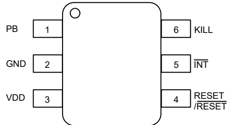
图 5-4. 引脚配置选项 TPS3424 DRL 封装 6 引脚 SOT-23 顶视图
