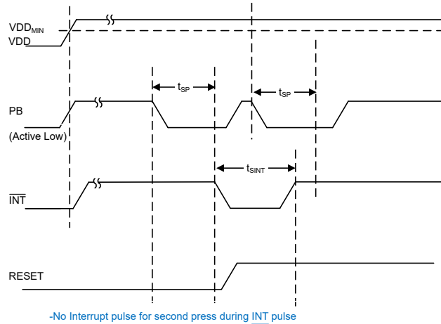
图 6-2. 时序图：PB 输入忽略示例
