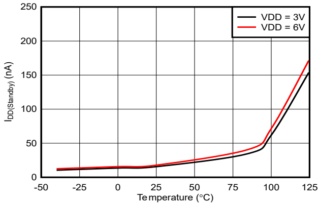
图 6-6. 待机电源电流与温度间的关系
