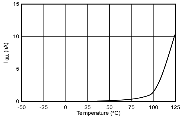
图 6-9. KILL 电流与温度间的关系
