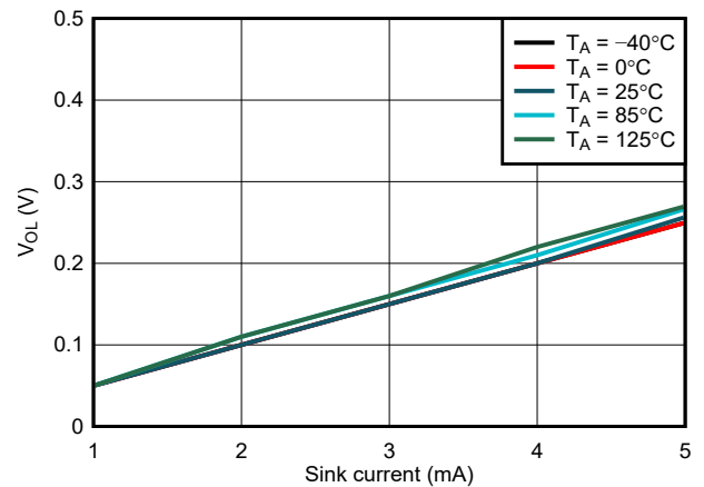
图 6-7. WDO V_{OL} 与 I_{sink} 间的关系, V_{DD} = 3.3V
