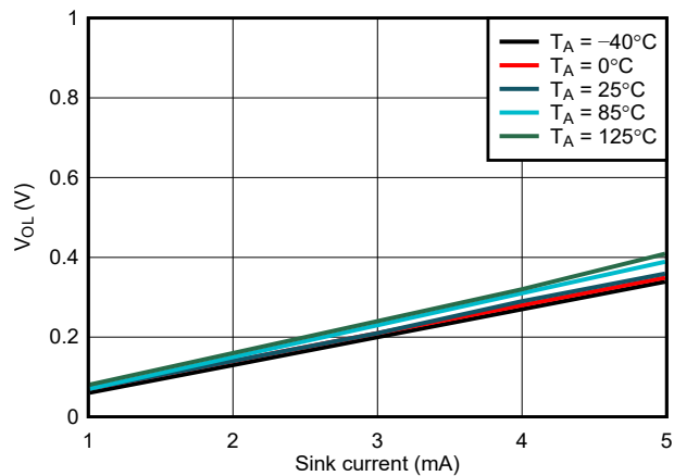
图 6-6. WDO V_{OL} 与 I_{sink} 间的关系, V_{DD} = 1.5V
