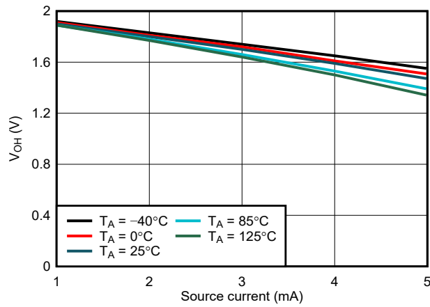
图 6-14. RESET V_{OH} 与 I_{source} 间的关系, V_{DD} = 2.0\text{V}
