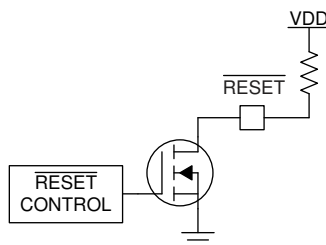
图 8-2. 开漏 RESET 配置
