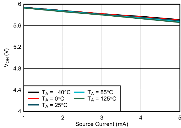
图 6-16. RESET V_{OH} 与 I_{source} 间的关系, V_{DD} = 6.0\text{V}
