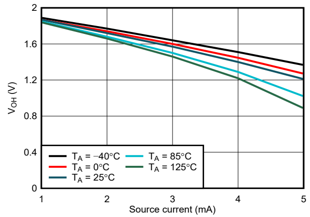
图 6-15. WDO V_{OH} 与 I_{source} 间的关系, V_{DD} = 2.0\text{V}
