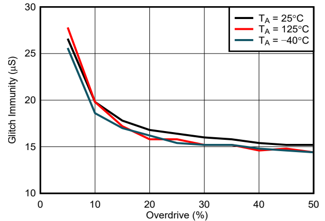
图 6-5. 电源抗干扰能力与过驱间的关系
