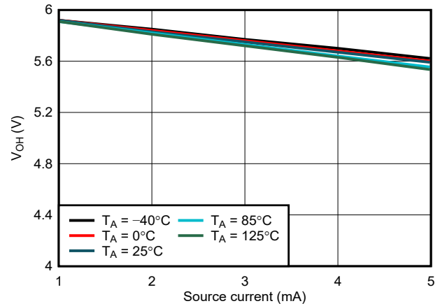
图 6-17. WDO V_{OH} 与 I_{source} 间的关系, V_{DD} = 6.0\text{V}
