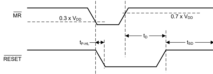
图 7-14. \overline{\text{MR}} 引脚响应
