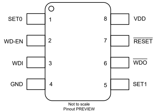
图 5-4. 引脚配置选项 D DDF 封装，8 引脚 SOT-23， TPS35 顶视图
