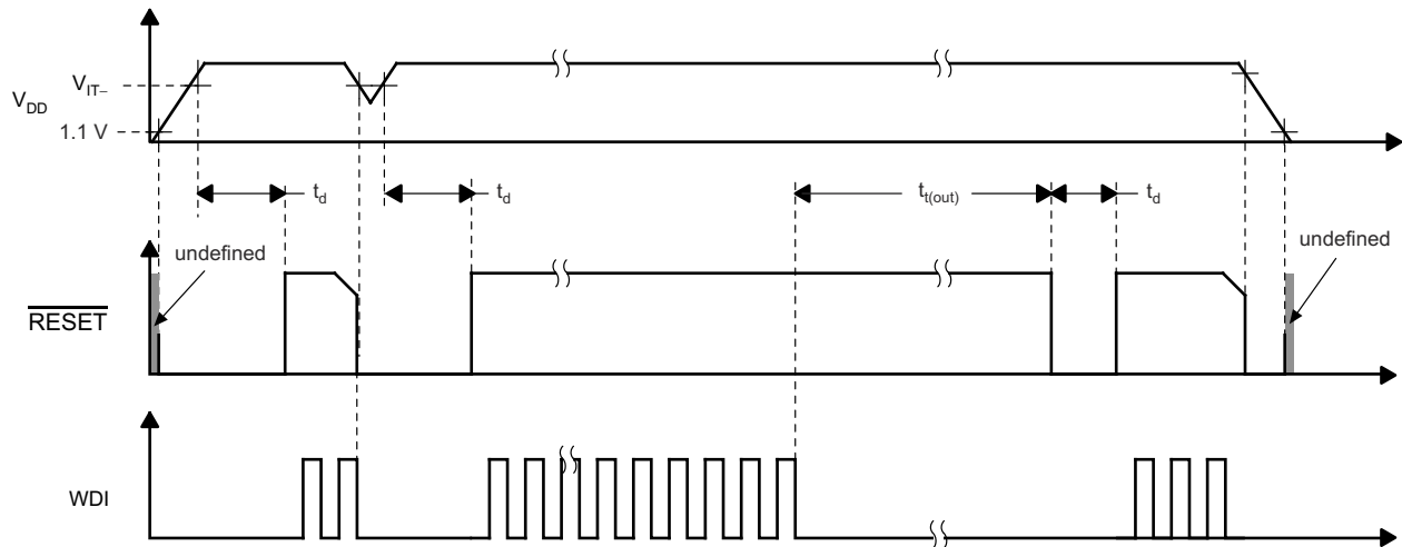
图 6-1. 时序图
