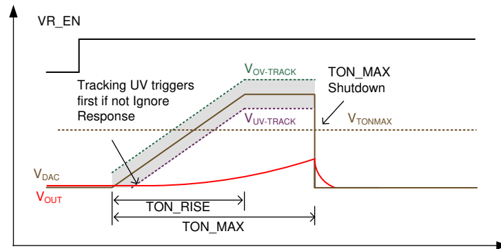
图 7-29. TON_MAX fault
