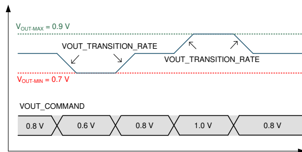
图 7-30. VOUT_MIN_MAX example
