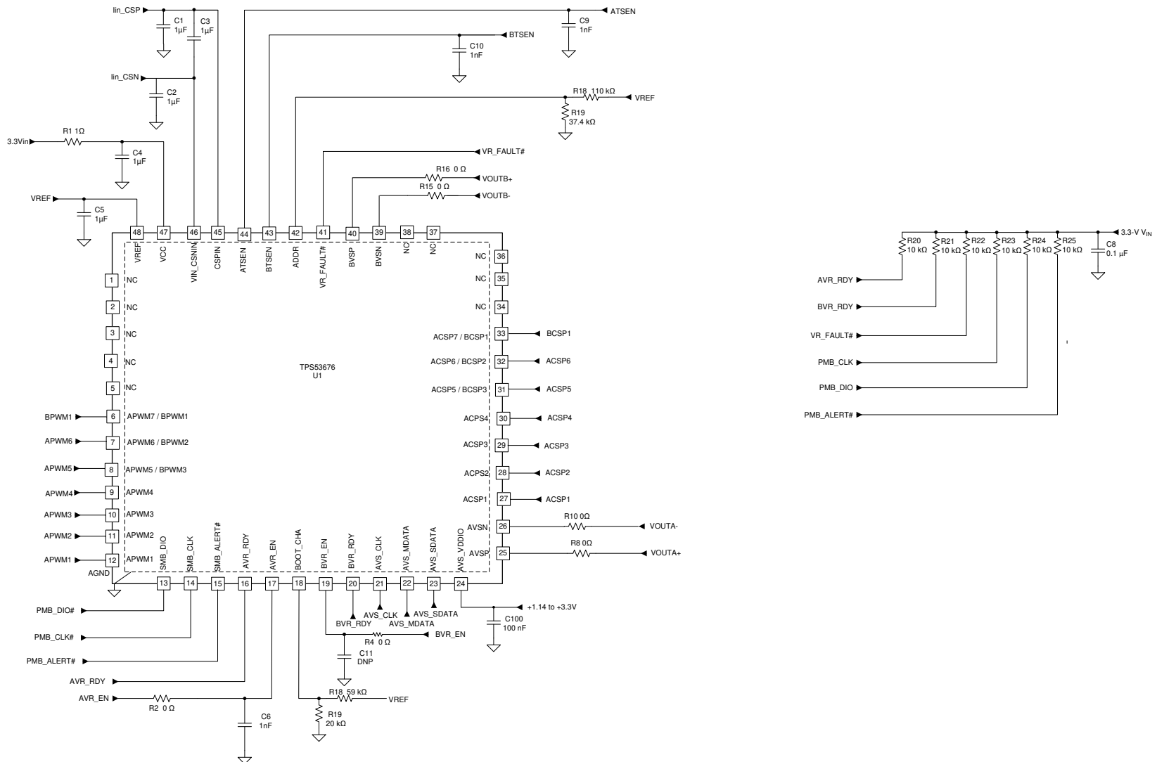
图 8-1. Controller Schematic
