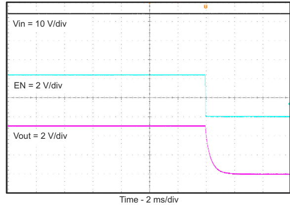
图 7-15. 相对于 EN 的关断
