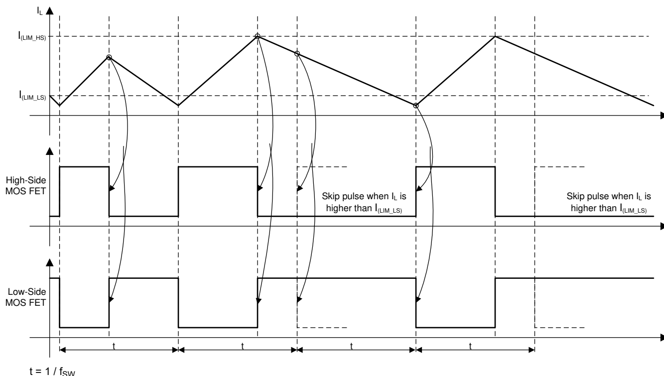
图 6-2. 针对两个 MOSFET 的过流保护
