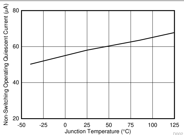
图 5-2. 非开关工作静态电流与结温间的关系
