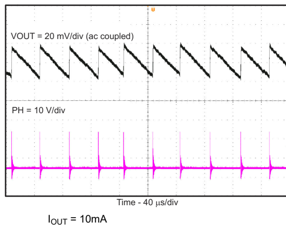
图 7-7. 输出电压纹波
