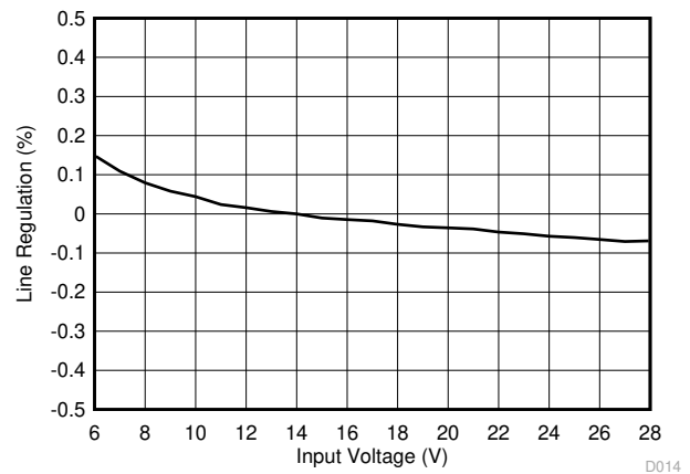
图 7-3. 线性调整率
