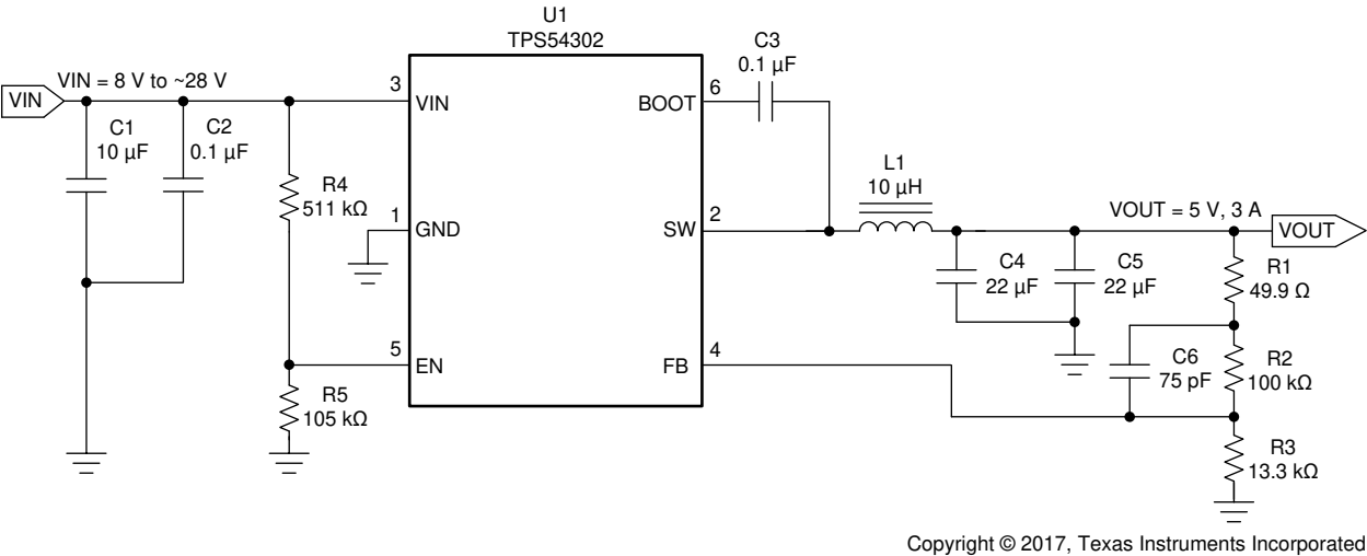
图 7-1. 5V、3A 参考设计
