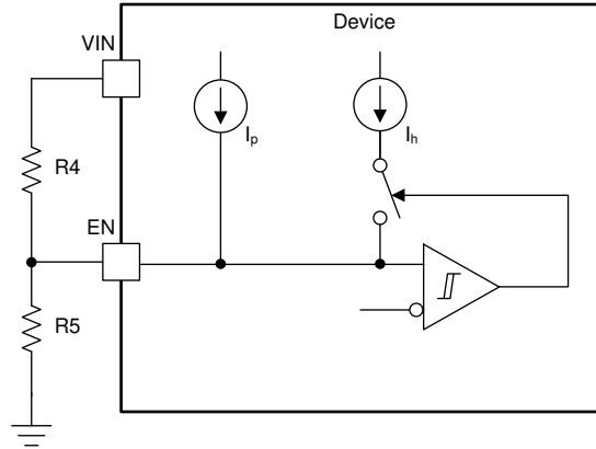
图 6-1. 可调节 VIN 欠压锁定
