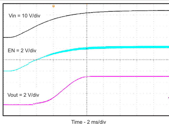
图 7-12. 相对于 VIN 的启动
