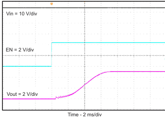
图 7-14. 相对于 EN 的启动
