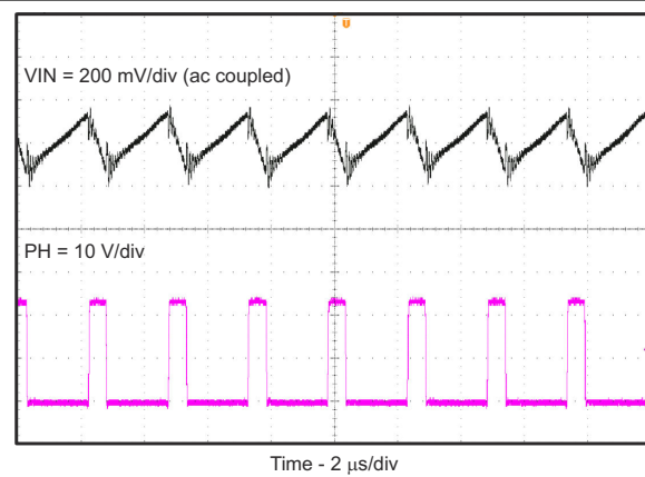
图 7-5. 输入电压纹波
