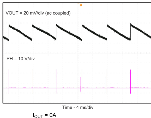
图 7-6. 输出电压纹波
