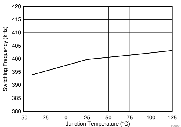
图 5-6. 中心开关频率与结温间的关系
