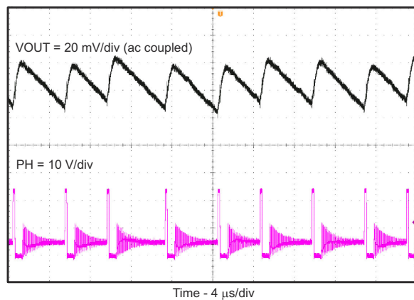
图 7-8. 输出电压纹波
