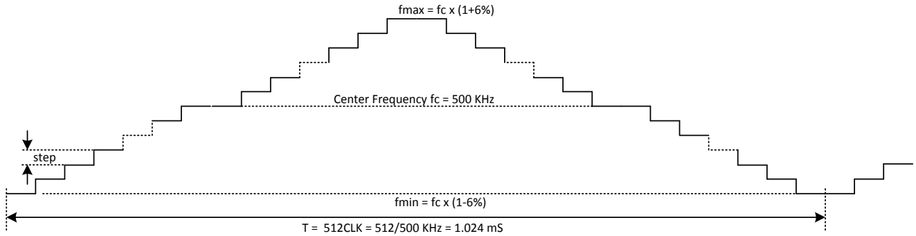
图 6-3. 展频频谱图
