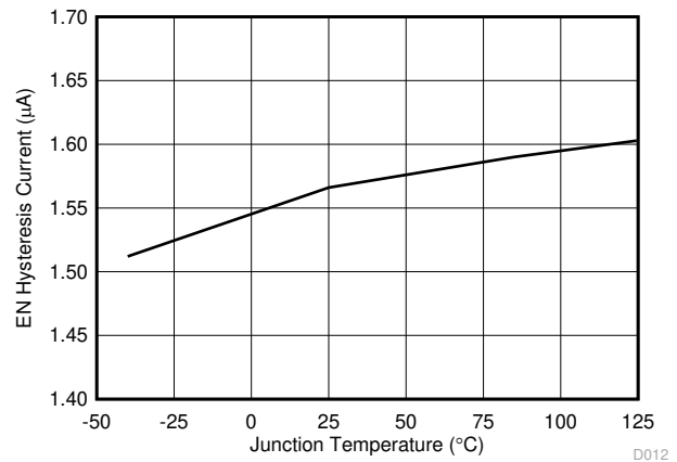
图 5-12. EN 迟滞电流与结温间的关系
