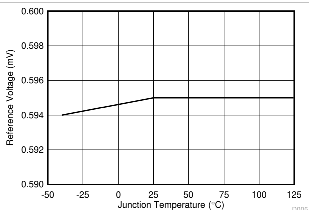
图 5-5. 基准电压与结温间的关系
