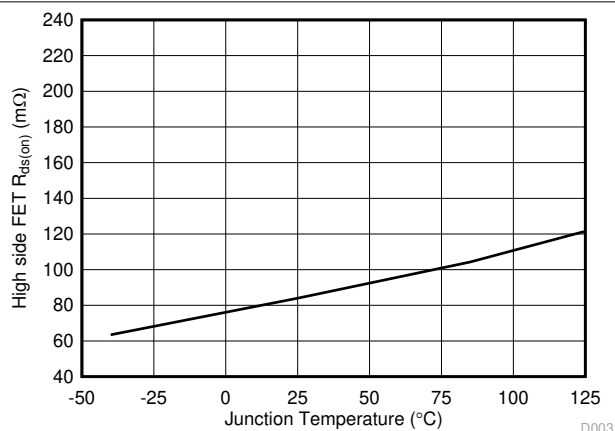
图 5-3. 高侧电阻与结温间的关系
