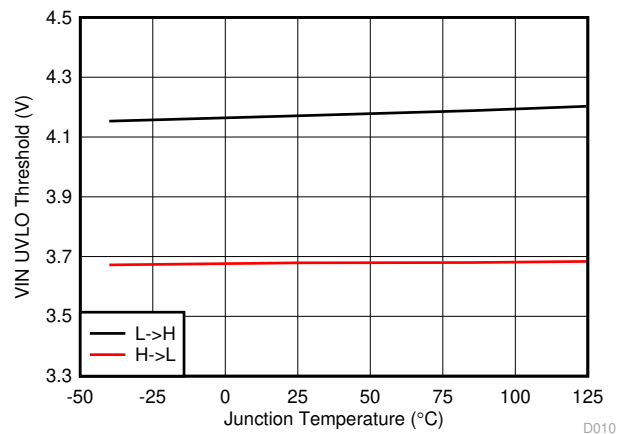
图 5-10. VIN UVLO 阈值与结温间的关系
