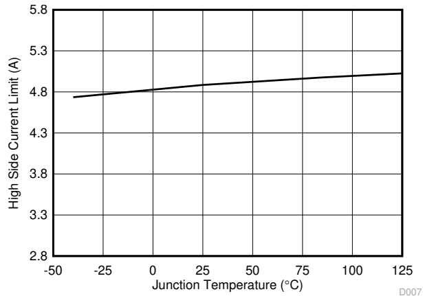
图 5-7. 高侧电流限制阈值与结温间的关系
