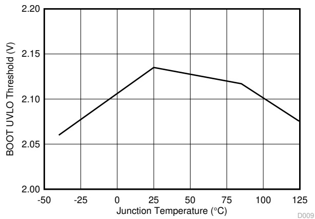
图 5-9. BOOT-SW UVLO 阈值与结温间的关系
