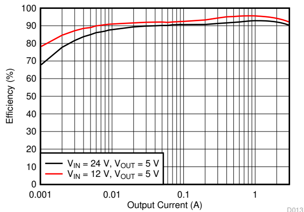
图 7-2. 效率
