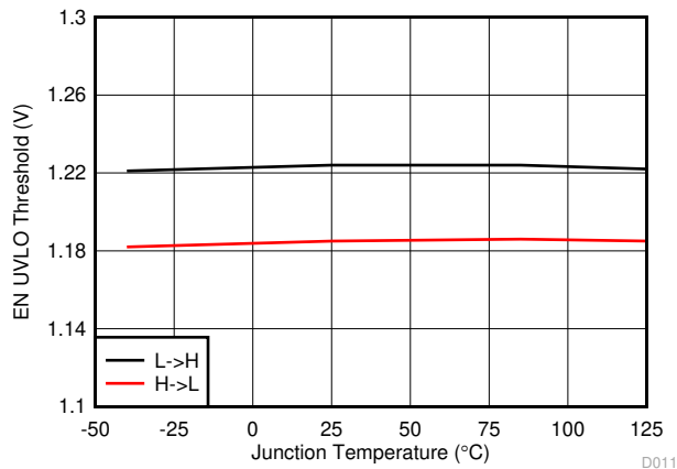
图 5-11. EN 阈值与结温间的关系
