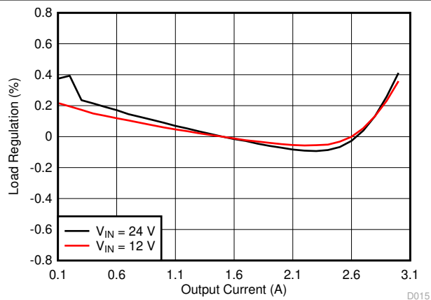
图 7-4. 负载调整率
