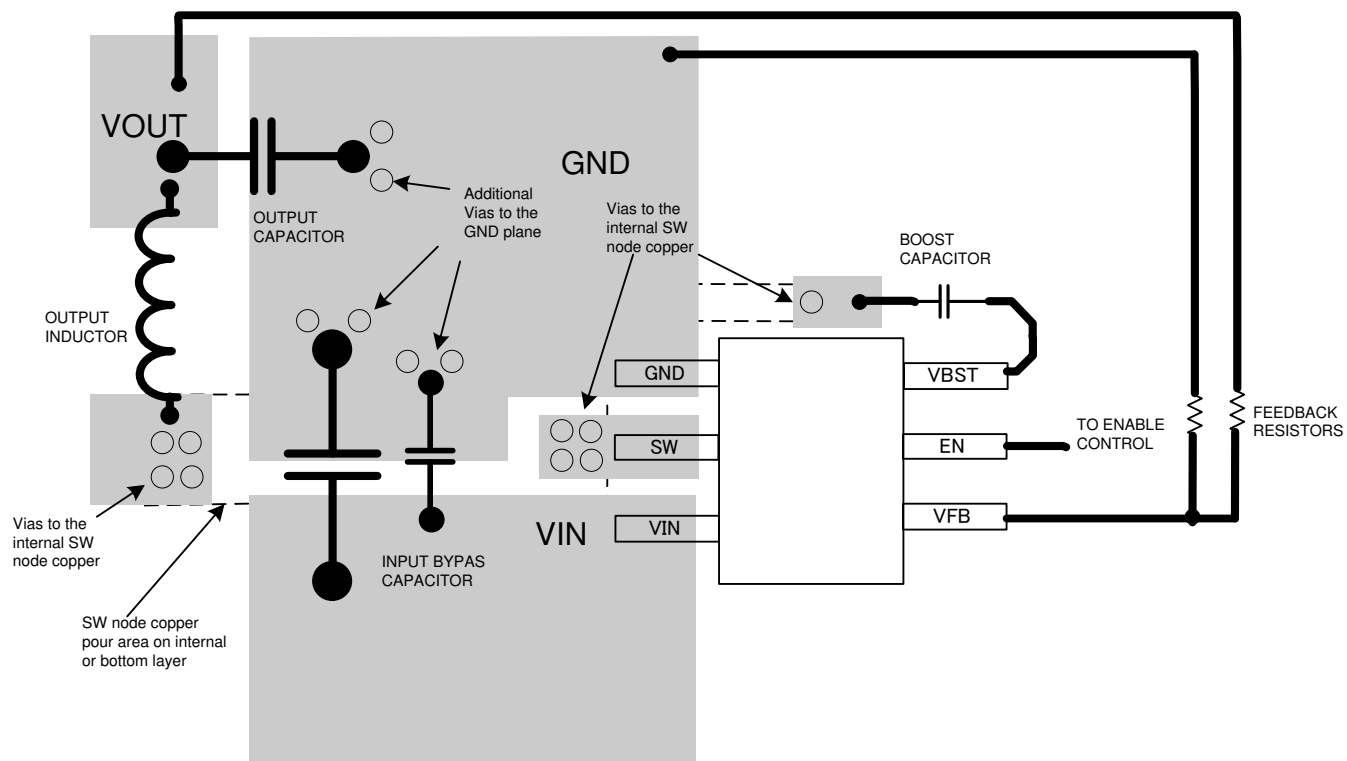
图 7-16. 电路板布局
