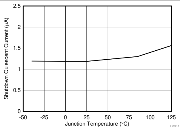
图 5-1. 关断静态电流与结温间的关系
