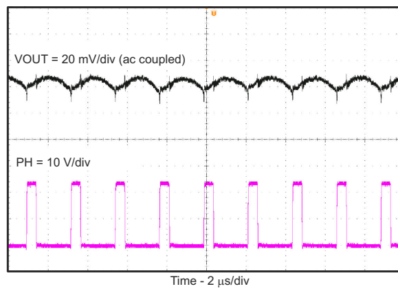
图 7-9. 输出电压纹波
