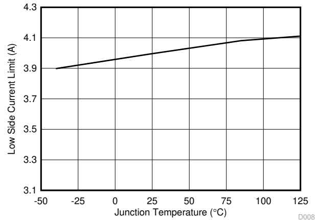
图 5-8. 低侧电流限制阈值与结温间的关系
