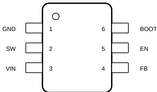
图 4-1. DDC 封装 6 引脚 SOT-23-THIN (顶视图)
