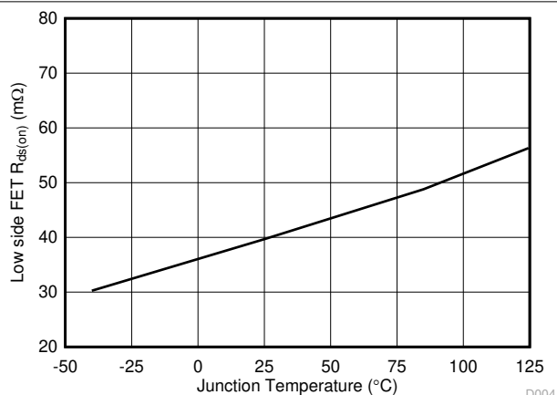
图 5-4. 低侧 FET 导通电阻与结温间的关系
