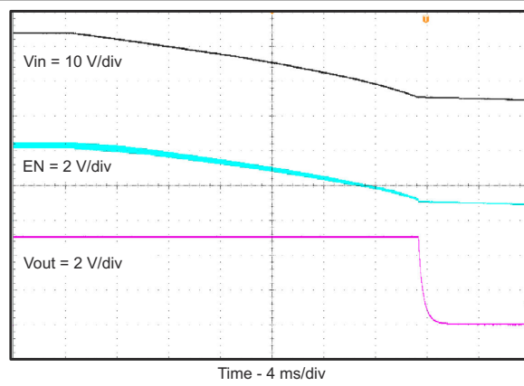
图 7-13. 相对于 VIN 的关断
