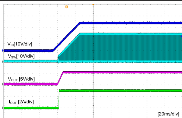
图 7-10. 由 V_{IN} 启动
