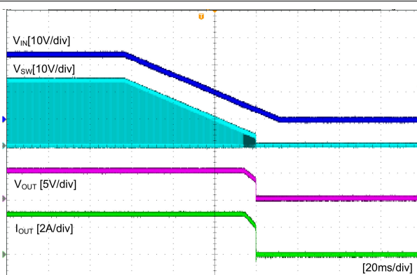
图 7-11. 依据 V_{IN} 的关断
