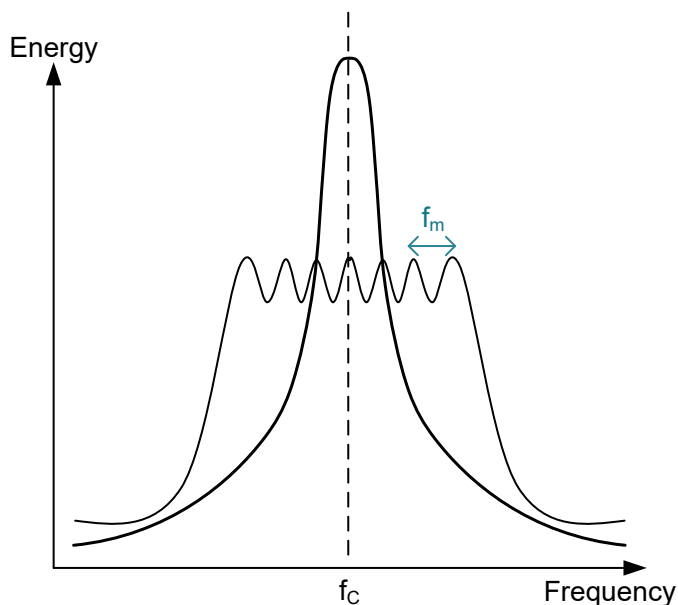
图 6-8. 能量与频率间的关系
