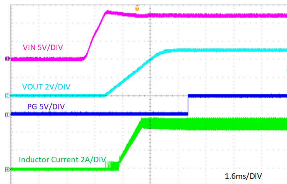
图 7-6. 相对于 V_{IN} 、 I_{OUT} = 5A 的启动
