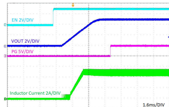
图 7-7. 通过 EN 的启动, I_{OUT} = 5A
