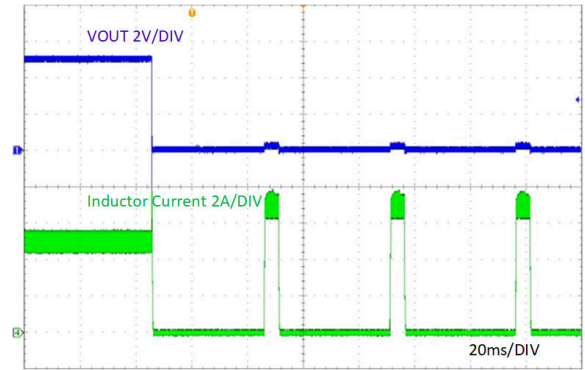
图 7-11. V_{OUT} 硬短路保护
