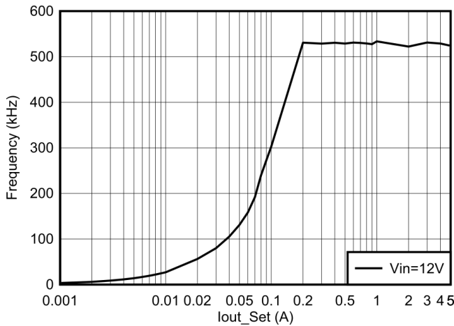
图 7-4. 开关频率与负载电流间的关系
