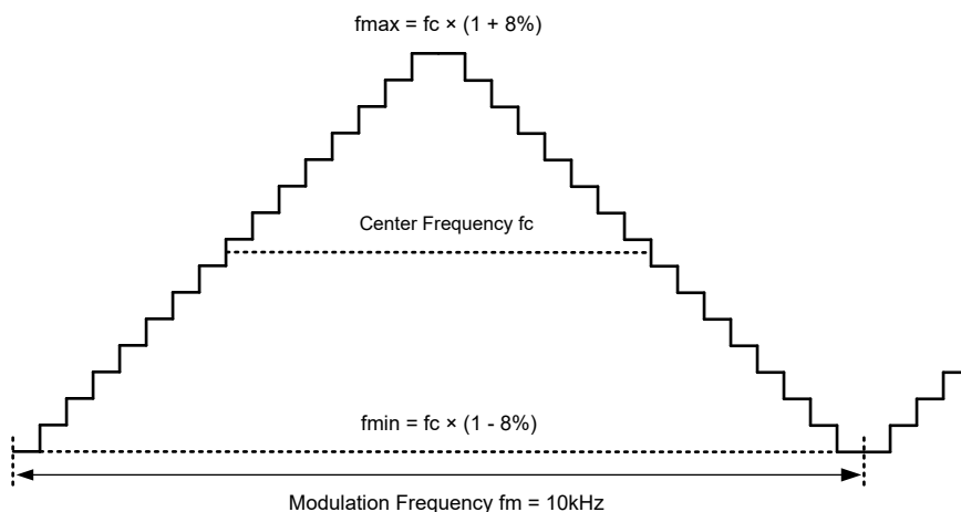
图 6-7. 展频频谱图
