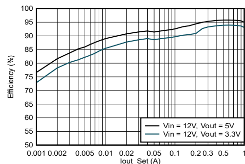
TPS542521 效率 ( V_{IN} = 12V , f_{SW} = 500kHz )
