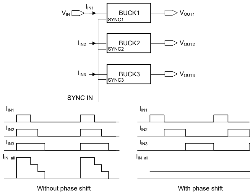
图 6-5. 相移操作应用
