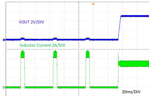
图 7-12. V_{OUT} 硬短路恢复
