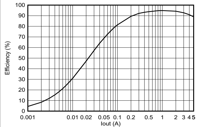
图 5-16. TPS543521 效率(FCCM), V_{IN} = 12\text{V} 、 V_{OUT} = 3.3\text{V} 、 f_{SW} = 500\text{kHz} 、 L = 4.7\mu\text{H}
