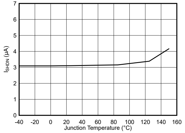
图 5-2. TPS543521 关断电流与结温间的关系
