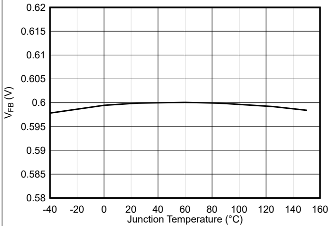
图 5-5. 反馈电压与结温间的关系
