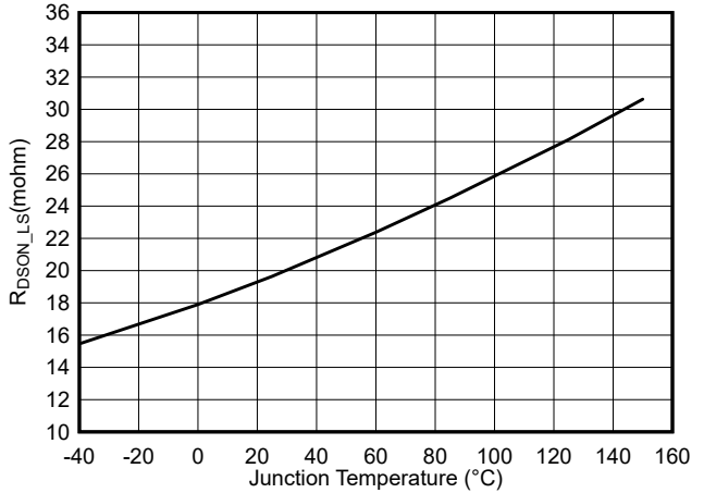
图 5-4. 低侧 R_{DS(on)} 与结温间的关系
