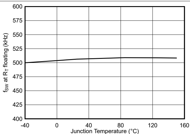
图 5-10. 开关频率 ( R_T 悬空) 与结温间的关系
