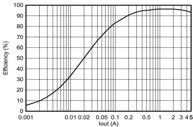
图 7-2. 效率 (FCCM)
