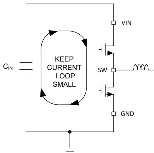
图 7-13. 具有快速边沿的电流环路
