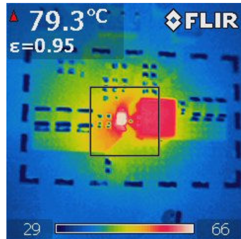
图 7-5. 外壳温度, V_{IN} = 12V , I_{OUT} = 5A , f_{SW} = 500kHz
