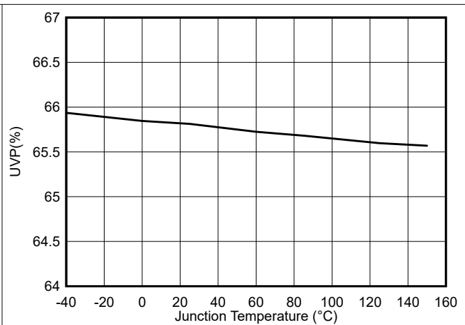
图 5-14. UVP 阈值与结温间的关系
