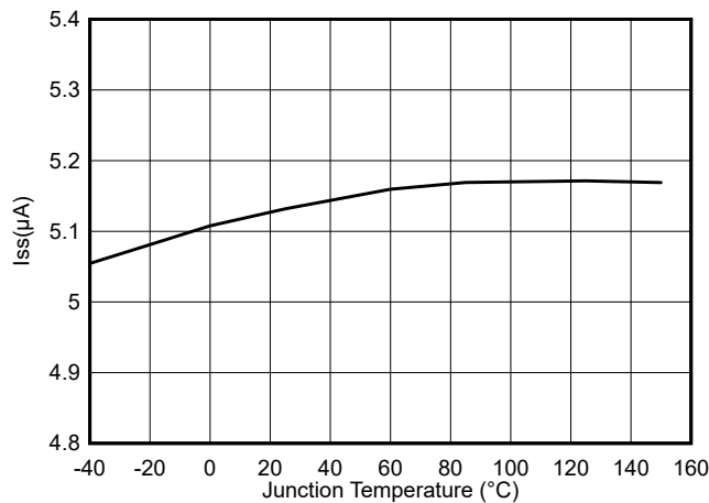
图 5-15. 软启动充电电流与结温间的关系
