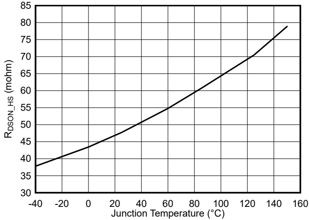
图 5-3. 高侧 R_{DS(on)} 与结温间的关系
