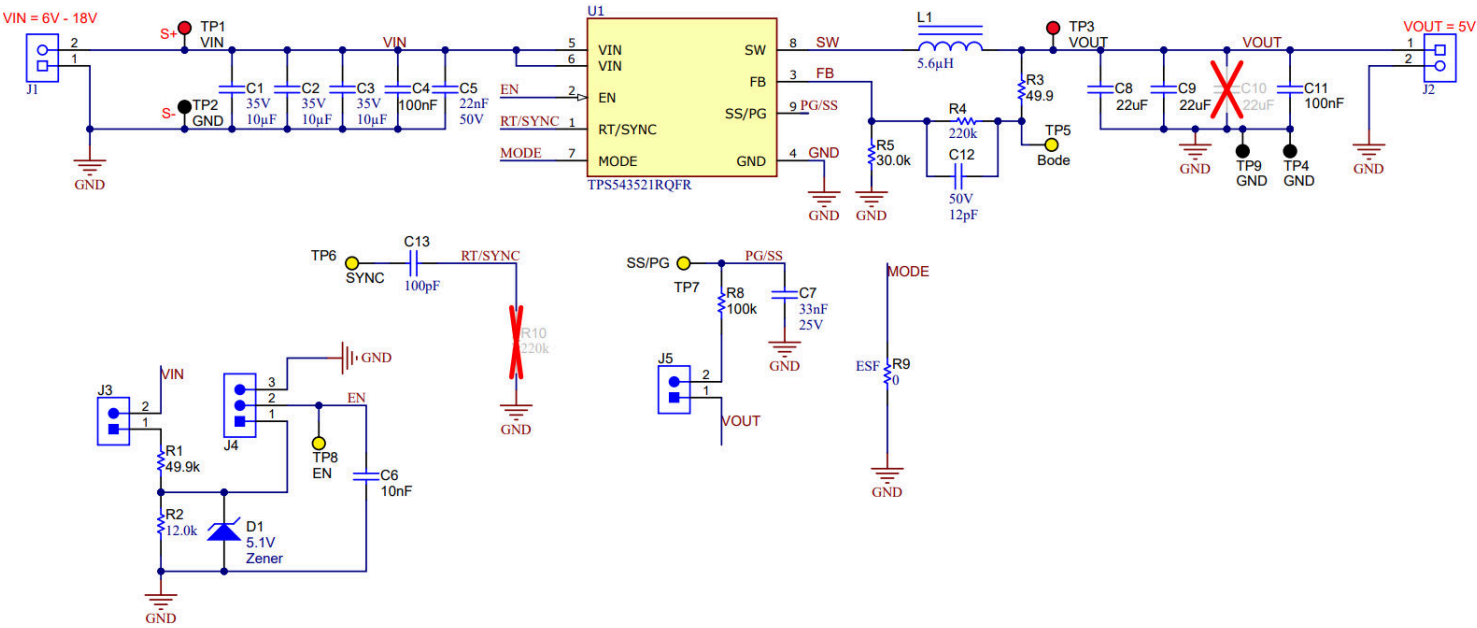
图 7-1. TPS543521 5V 输出、5A 参考设计
