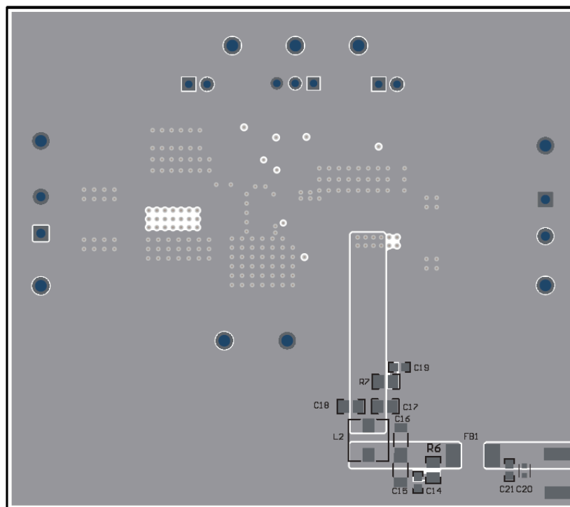
图 7-15. TPS543521 底层布局示例
