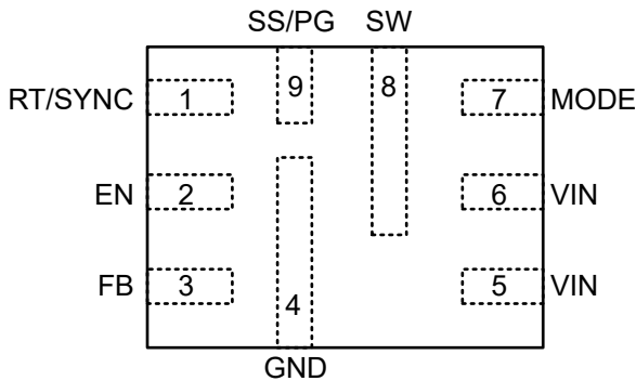
图 4-1. 9 引脚 RQF VQFN-HR , 1.5mm × 2mm 封装 ( 顶视图 )
