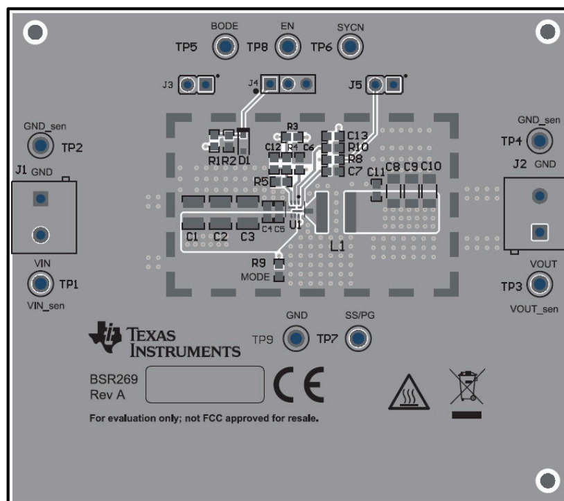
图 7-14. TPS543521 顶层布局示例
