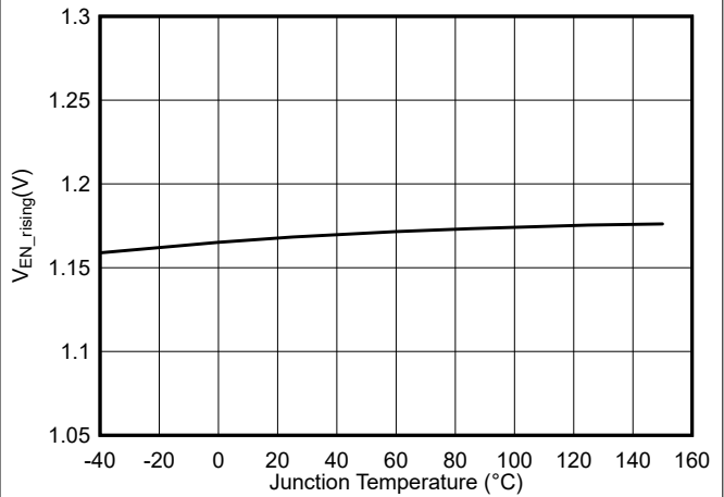
图 5-6. 启用阈值与结温间的关系
