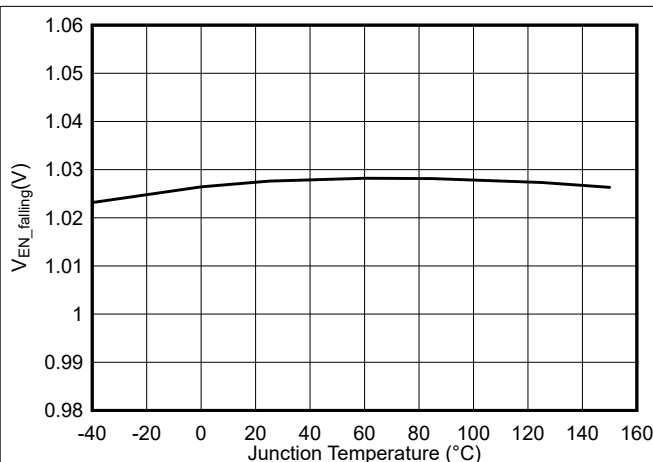
图 5-7. 禁用阈值与结温间的关系
