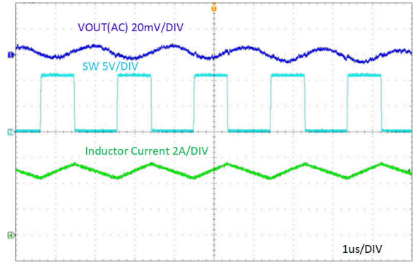
图 7-9. 稳态, I_{OUT} = 5A
