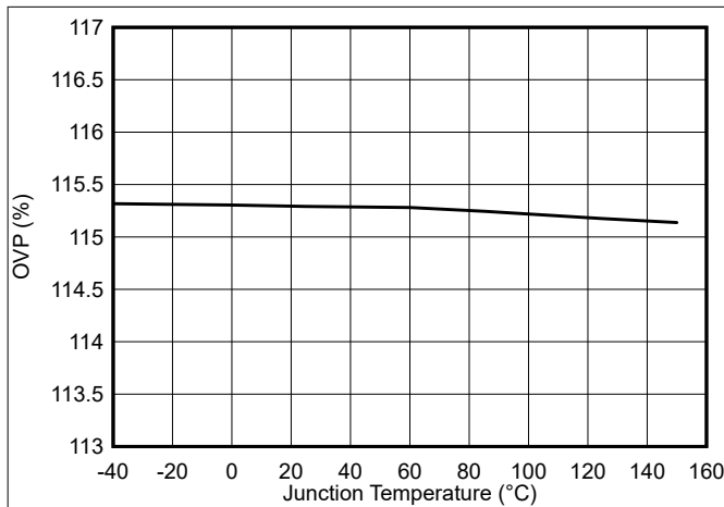
图 5-13. OVP 阈值与结温间的关系
