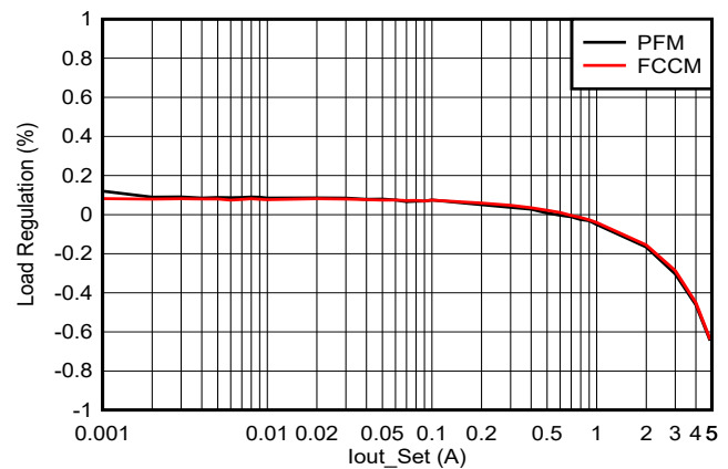
图 7-3. 负载调整率
