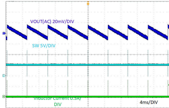
图 7-8. 稳态, I_{OUT} = 0A
