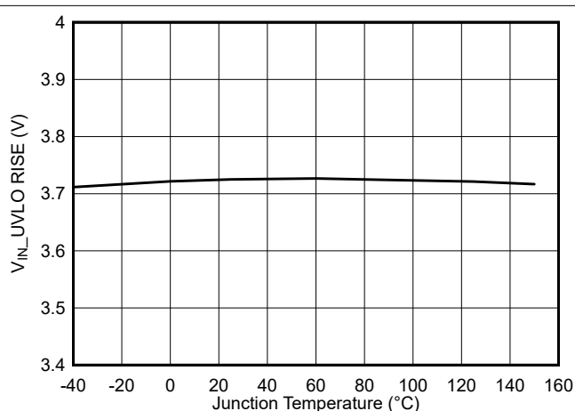
图 5-8. V_{IN} UVLO 上升阈值与结温间的关系
