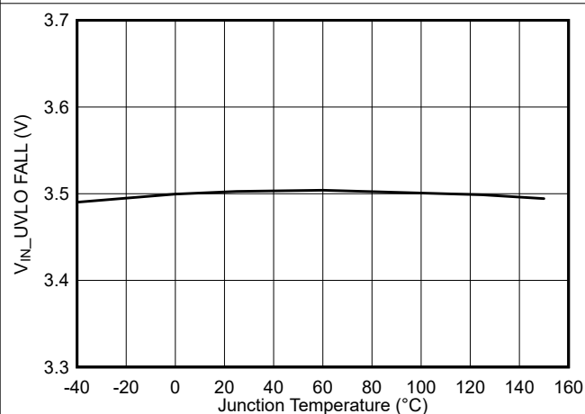
图 5-9. V_{IN} UVLO 下降阈值与结温间的关系
