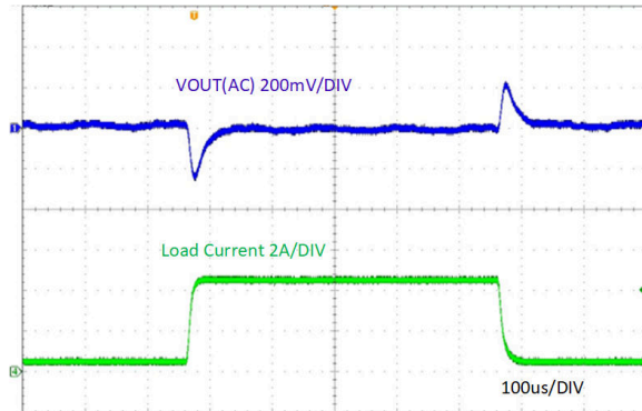
图 7-10. 负载瞬态响应, 0.5A 至 4.5A, 压摆率 = 0.8A/ \mu S
