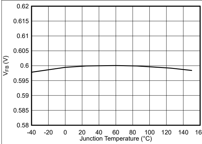
图 5-5. 反馈电压与结温间的关系
