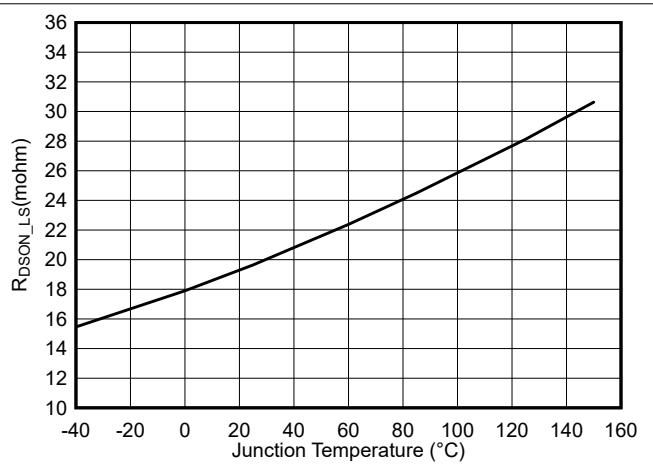
图 5-4. 低侧 R_{DS(on)} 与结温间的关系
