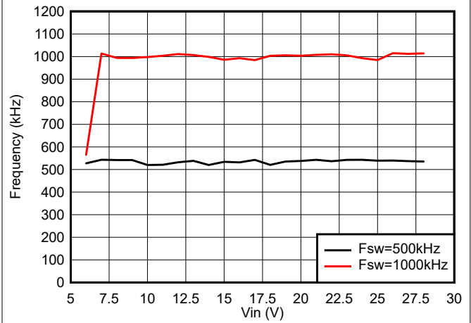
图 5-20. TPS54538 开关频率与 V_{IN} 间的关系, V_{OUT} = 5\text{V} , I_{OUT} = 5\text{A}
