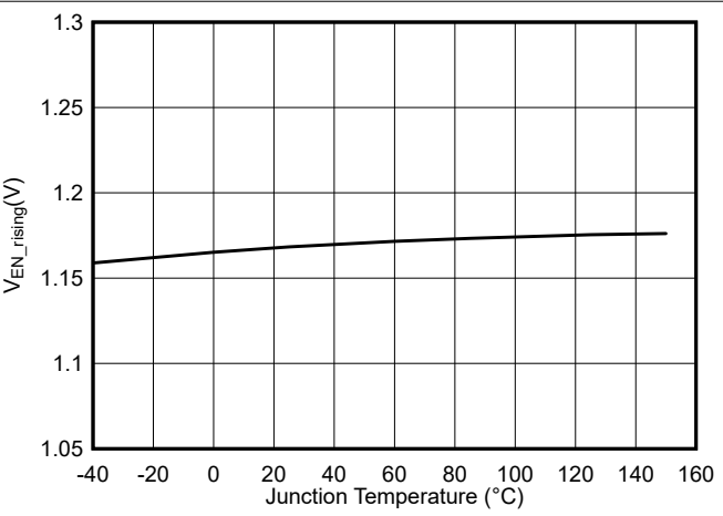
图 5-6. 启用阈值与结温间的关系
