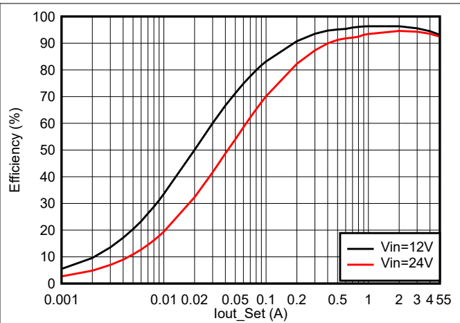
图 7-3. 效率 (FCCM)
