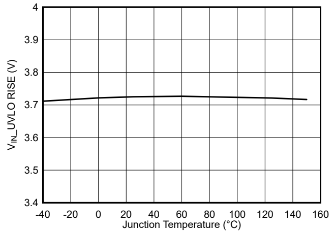
图 5-8. V IN UVLO 上升阈值与结温间的关系
