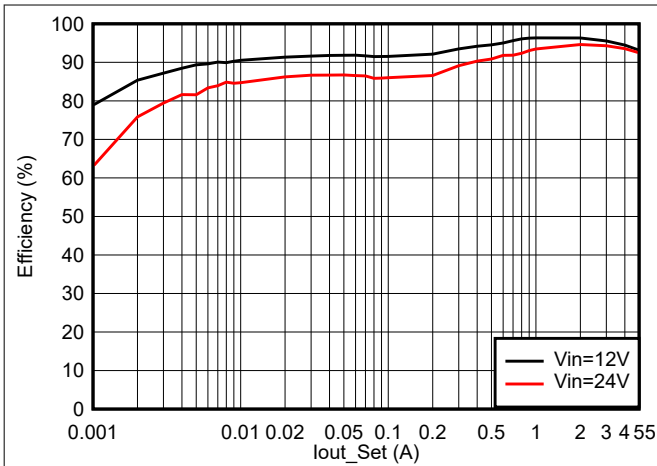
图 7-2. 效率 (PFM)
