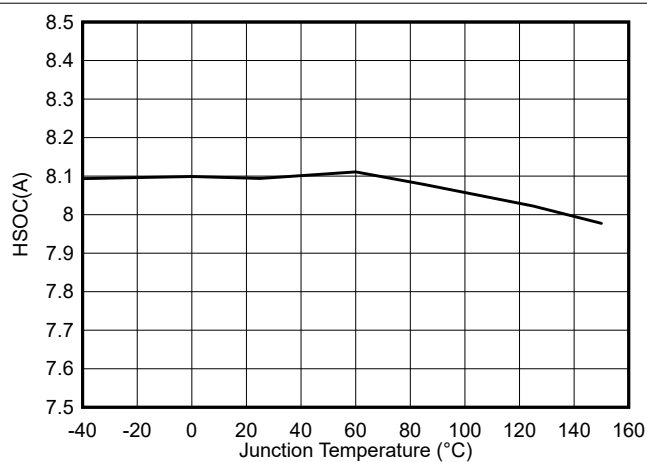
图 5-11. TPS54538 高侧电流限值与结温间的关系
