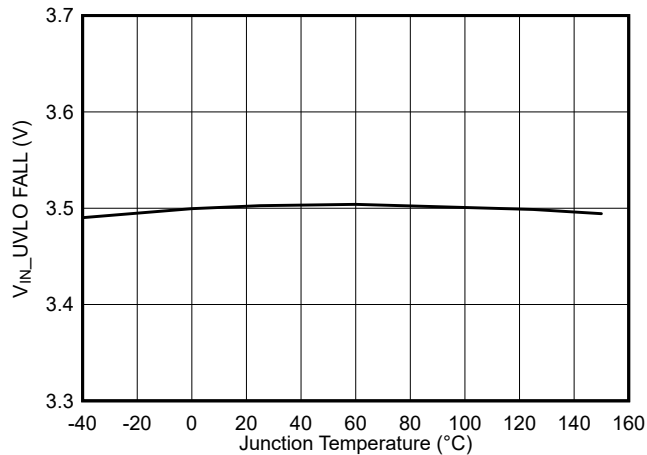
图 5-9. V IN UVLO 下降阈值与结温间的关系
