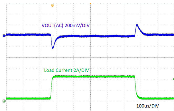
图 7-14. 负载瞬态响应，0.5A 至 4.5A，压摆率 = 0.8A/ \mu S
