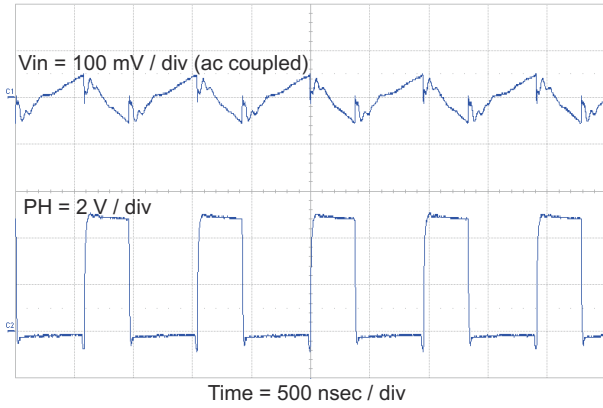
图 8-8. Input Ripple
