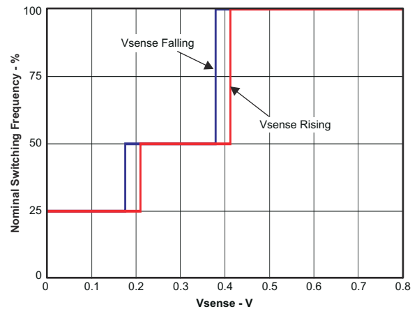
图 6-6. Switching Frequency vs Vsense
