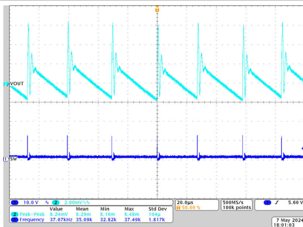
图 8-4. 输出电压纹波，1.2V Vout，800kHz DCM，空载
