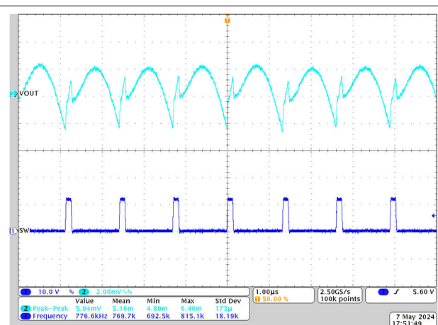
图 8-3. 输出电压纹波，1.2V Vout，800kHz FCCM，25A 负载
