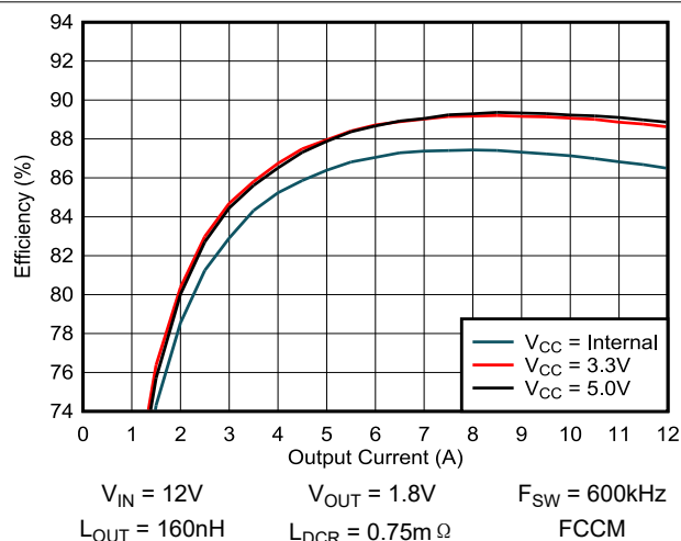
图 5-6. 效率与 V_{CC} 偏置之间的关系 ( V_{OUT} = 1.8V )
