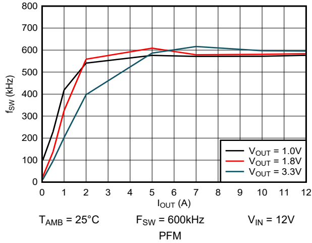
图 5-23. 开关频率与输出电流间的关系
