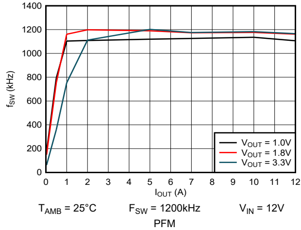
图 5-17. 开关频率与输出电流间的关系
