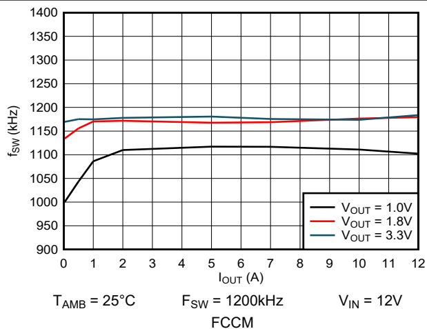
图 5-16. 开关频率与输出电流间的关系
