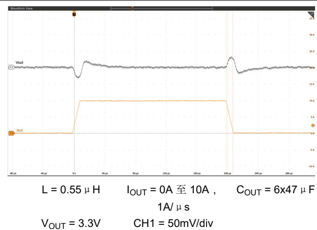
图 7-6. 负载瞬态
