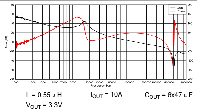
图 7-7. 频率响应
