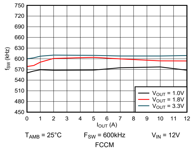
图 5-22. 开关频率与输出电流间的关系
