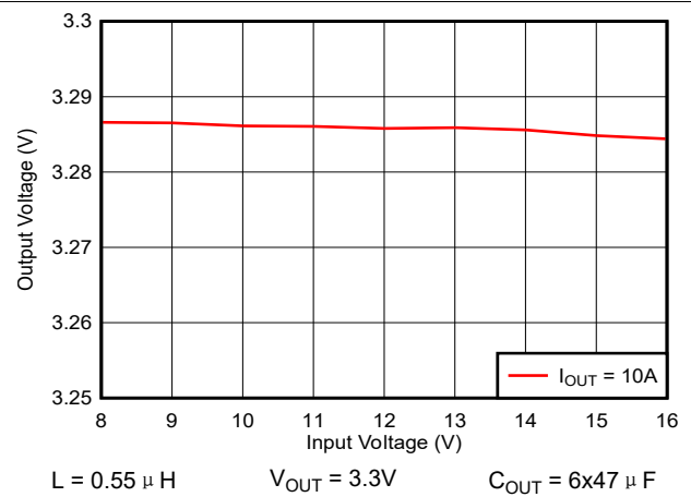
图 7-5. 线性调整率
