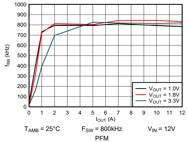
图 5-20. 开关频率与输出电流间的关系
