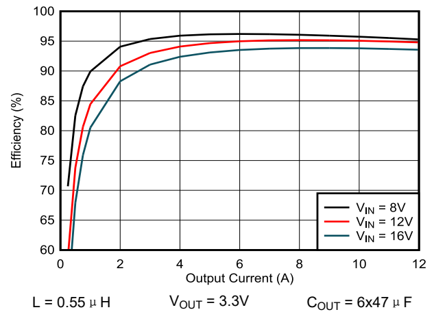
图 7-3. 效率 - FCCM 模式
