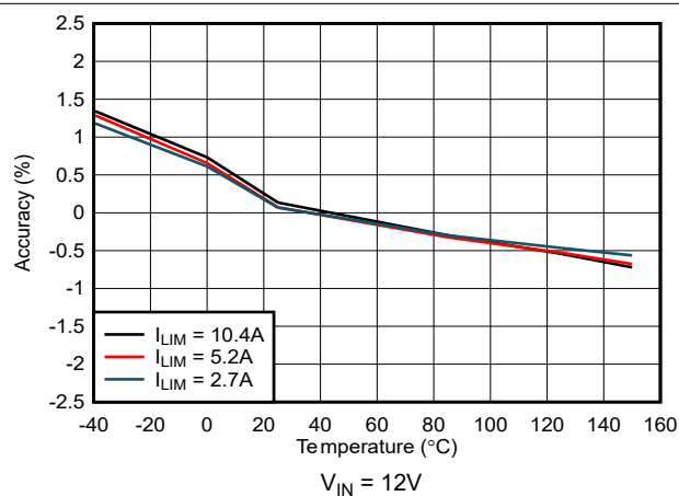
图 5-31. 低侧谷电流限制精度 (外部) 与结温间的关系
