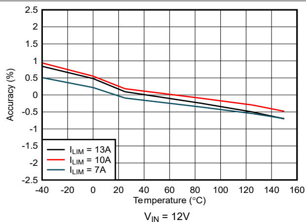
图 5-30. 低侧谷电流限制精度 (内部) 与结温间的关系
