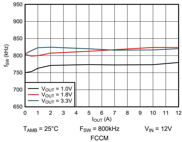
图 5-19. 开关频率与输出电流间的关系
