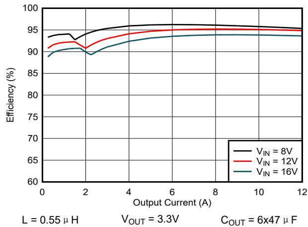
图 7-2. 效率 - PFM 模式
