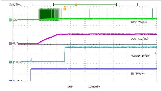
图 8-16. Enable Power Up, Skip
