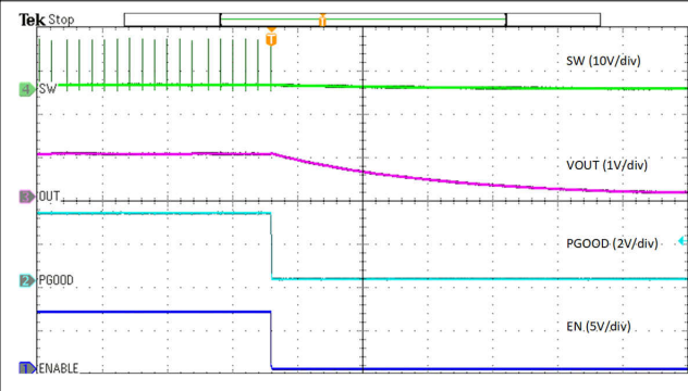
图 8-15. Prebias Power Down
