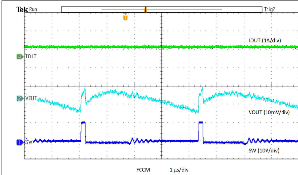
图 8-22. Output Voltage Ripple, FCCM, 0.5-A Load
