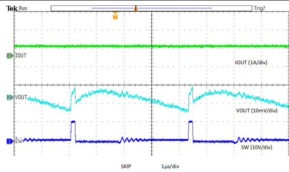
图 8-25. Output Voltage Ripple, Skip, 1-A Load
