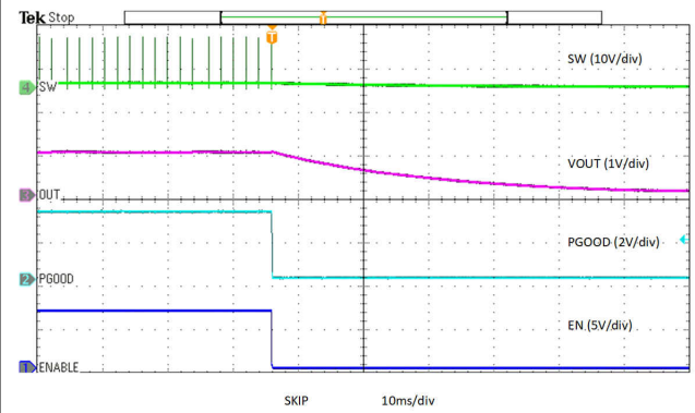
图 6-14. Enable Power Down, Skip
