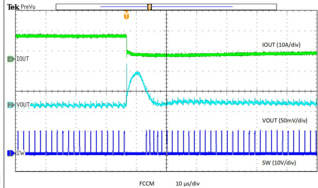
图 6-12. Unload Transient
