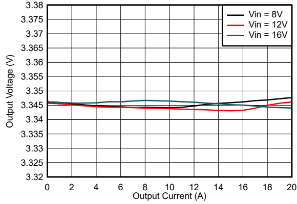
图 6-7. Output Voltage vs Output Current
