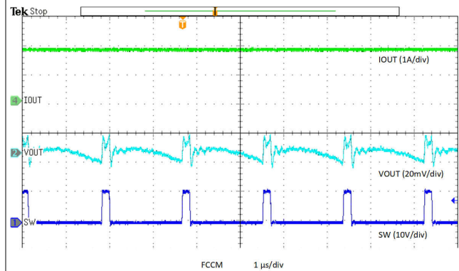
图 6-16. V_{OUT} Ripple, FCCM, 20-A Load
