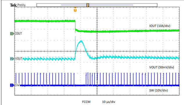
图 8-20. Unload Transient
