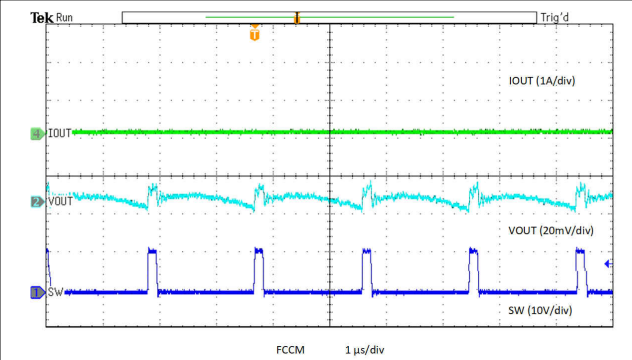
图 8-21. Output Voltage Ripple, FCCM, 0-A Load
