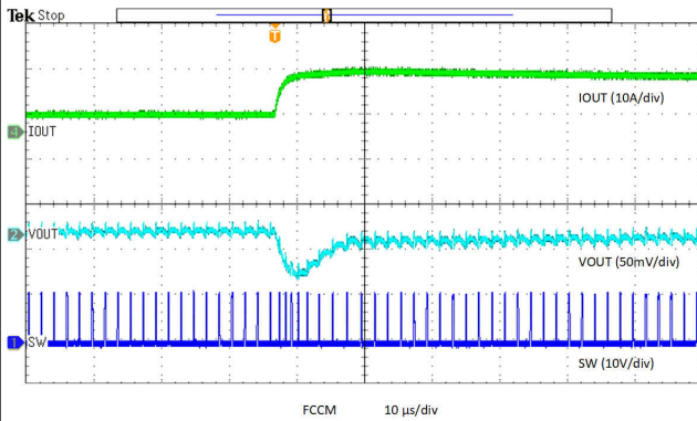
图 6-11. Load Transient
