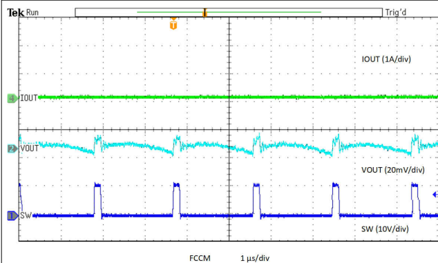
图 6-17. V_{OUT} Ripple, FCCM, 0-A Load
