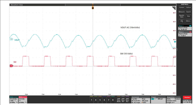
V_{IN} = 12V V_{OUT} = 3.3V I_{OUT} = 25A 图 7-9. 输出电压纹波 - FCCM
