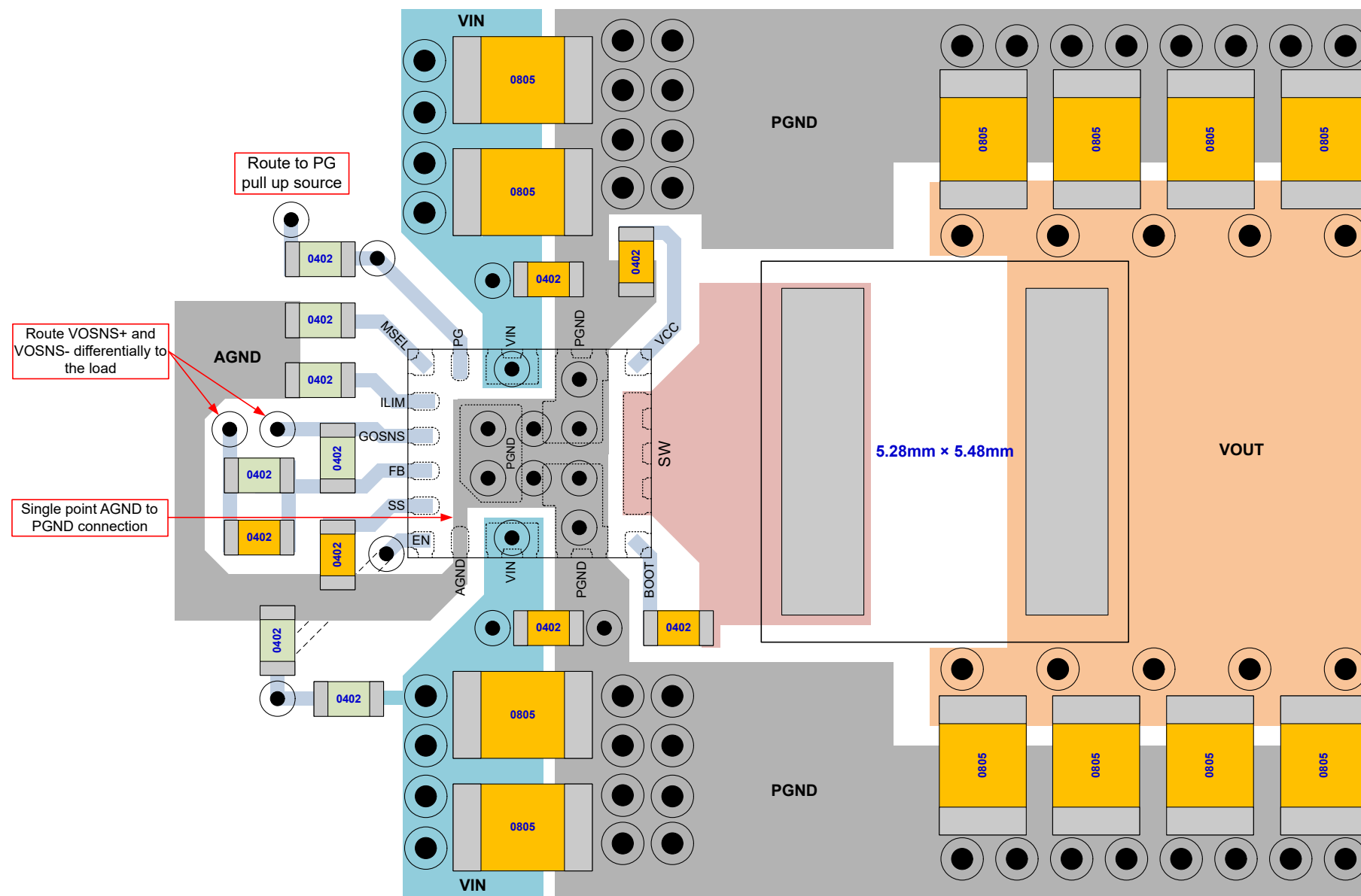
图 7-12. 布局建议
