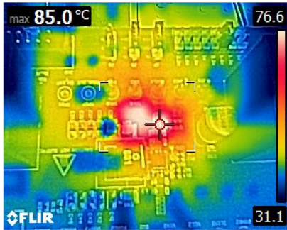
图 5-7. 热图像 - 5V 输出, TPS54KB20EVM, 6 层
