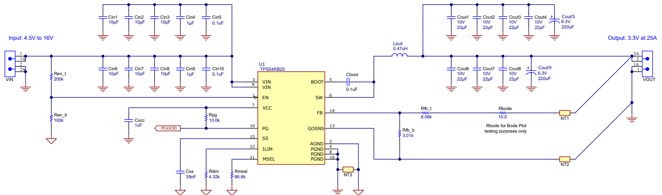
图 7-1. 应用电路图
