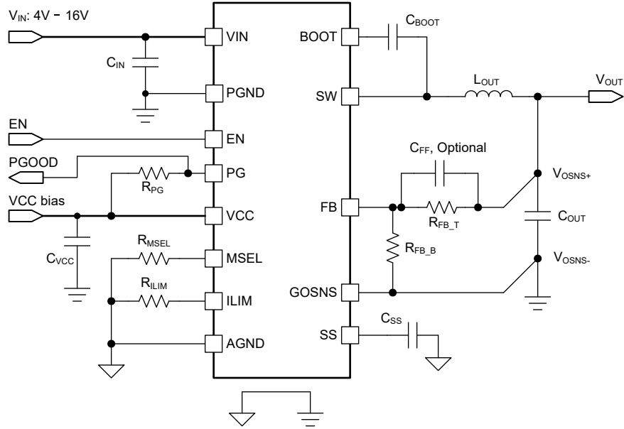
图 6-10. 具有外部 VCC 辅助电源的分离轨配置
