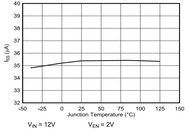
图 5-32. SS 引脚输出电流与结温间的关系
