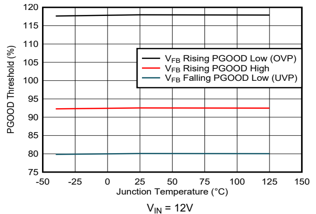
图 5-36. 电源正常阈值与结温的关系 ( V_{REF} = 0.9V )
