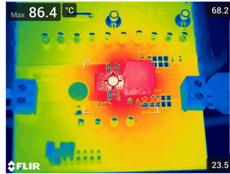
图 5-8. 热图像 - 3.3V 输出, TPS54KB20EVM, 6 层
