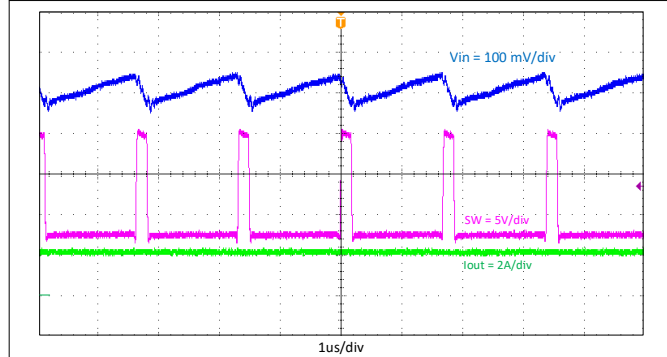
图 8-4. 输入电压纹波
