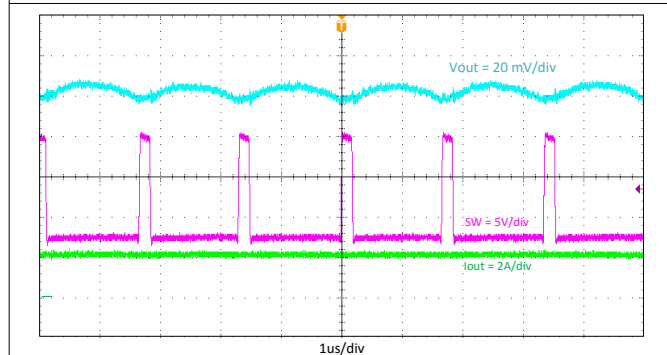
图 8-6. 输出电压纹波, I_{out} = 2A
