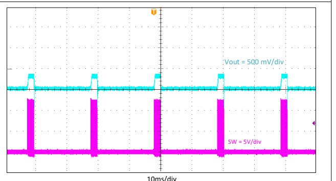
图 8-7. 断续, I_{out} = 5A
