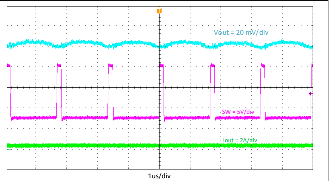
图 8-5. 输出电压纹波, I_{out} = 0.2A
