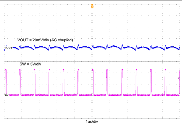
图 7-3. TPS562246 输出电压纹波 (0.01A 负载)
