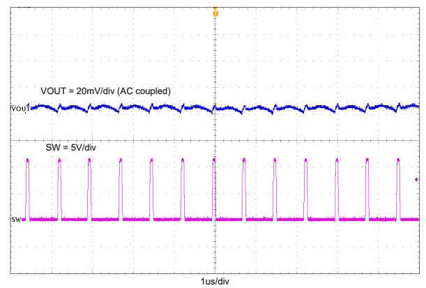
图 7-5. TPS562246 输出电压纹波 (2A 负载)
