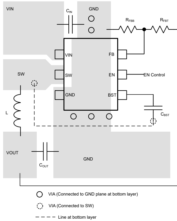
图 7-18. TPS56224x 布局
