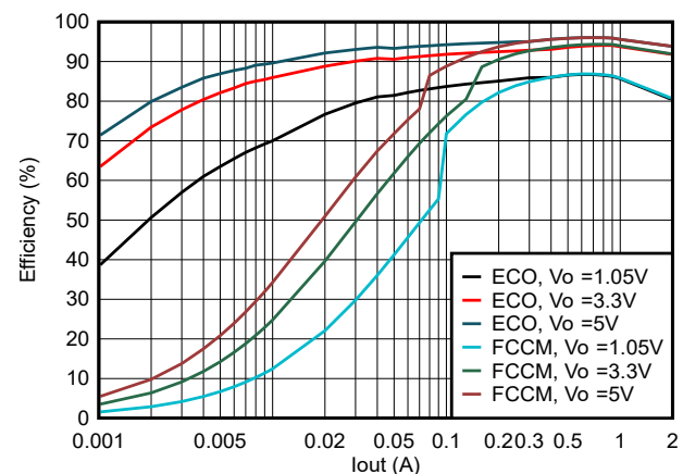
TPS56224x 在 Vin = 12V 时的效率
