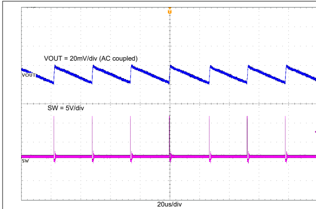
图 7-2. TPS562243 输出电压纹波 (0.01A 负载)
