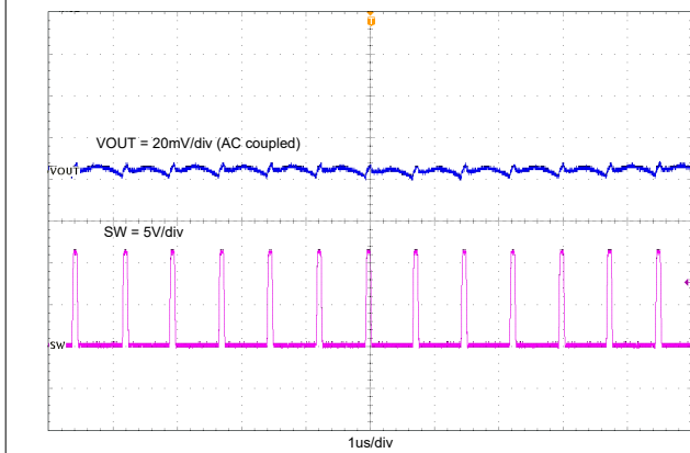
图 7-4. TPS562243 输出电压纹波 (2A 负载)
