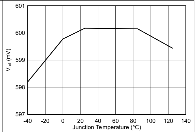
图 5-2. Vref 电压
