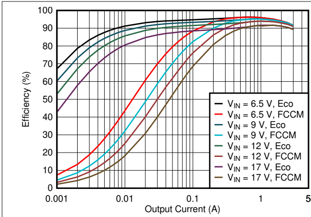
图 8-2. 效率
