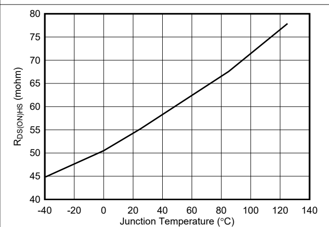
图 6-6. High-Side R_{DS(ON)}
