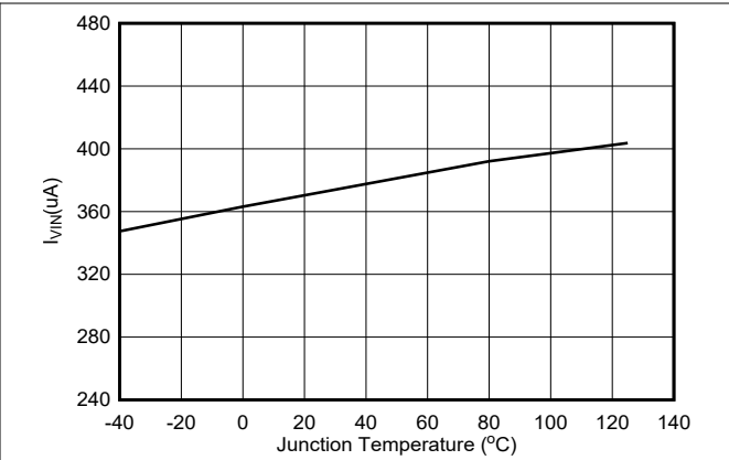
图 6-2. TPS563257 Quiescent Current
