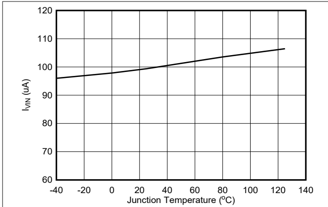
图 6-1. TPS563252 Quiescent Current
