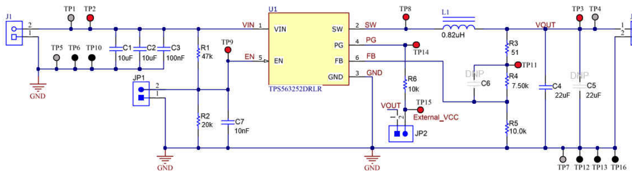
图 8-1. Schematic
