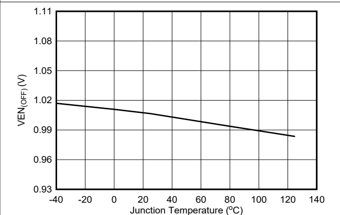
图 6-4. Enable Off Threshold Voltage
