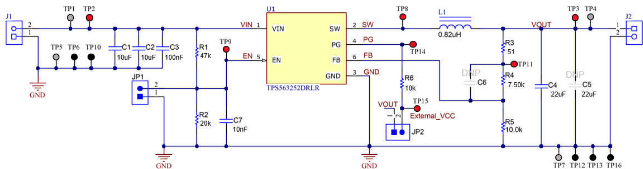
图 8-1. Schematic
