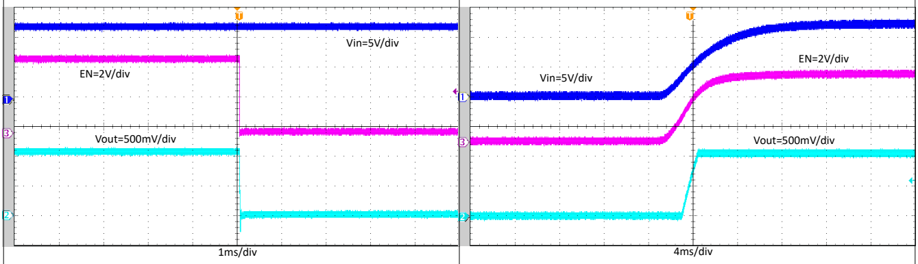
图 8-12. 通过 EN 关断, I_{OUT} = 4A
