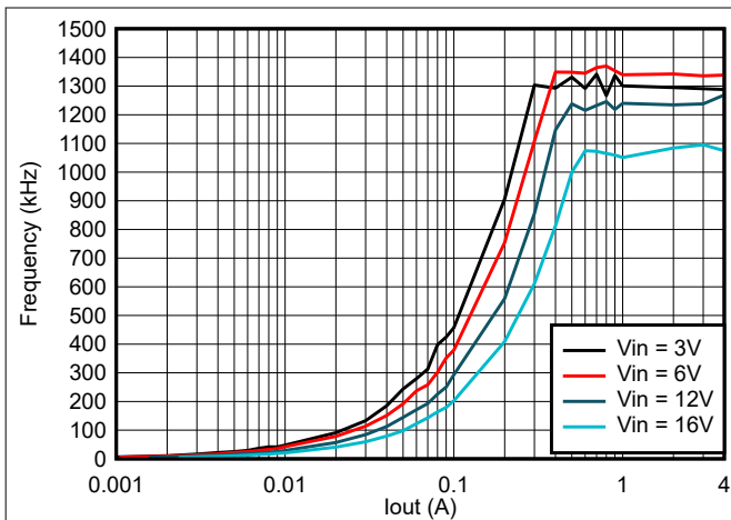
图 8-2. TPS564242 频率与负载间的关系
