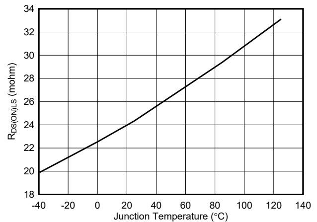
图 6-6. Low-Side R_{DS(ON)}
