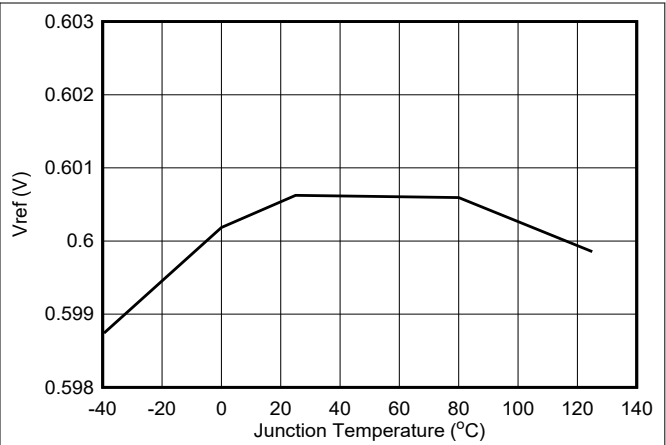
图 6-8. VREF Voltage
