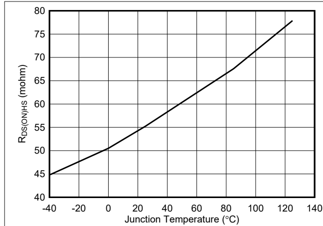
图 6-7. High-Side R_{DS(ON)}
