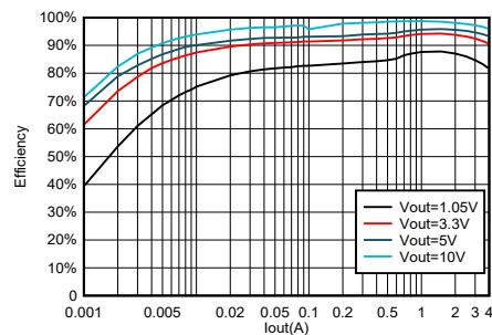
TPS564252 在 V_{IN} = 12V 时的效率
