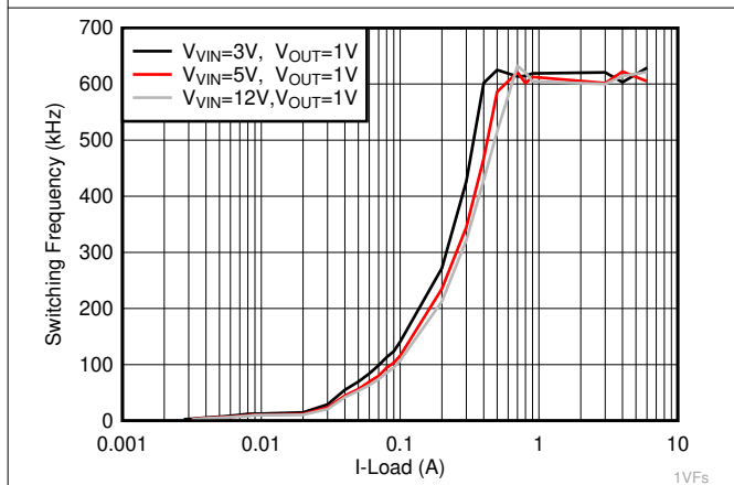
图 7-6. TPS566231 F_{SW} vs Output Load
