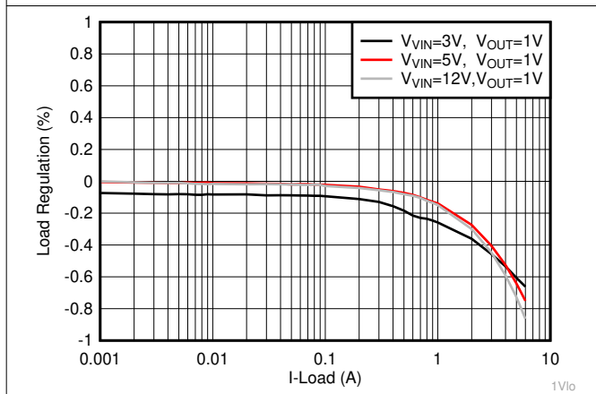
图 7-4. TPS566231 Load Regulation
