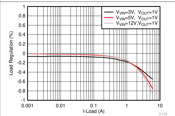
图 7-5. TPS566238 Load Regulation
