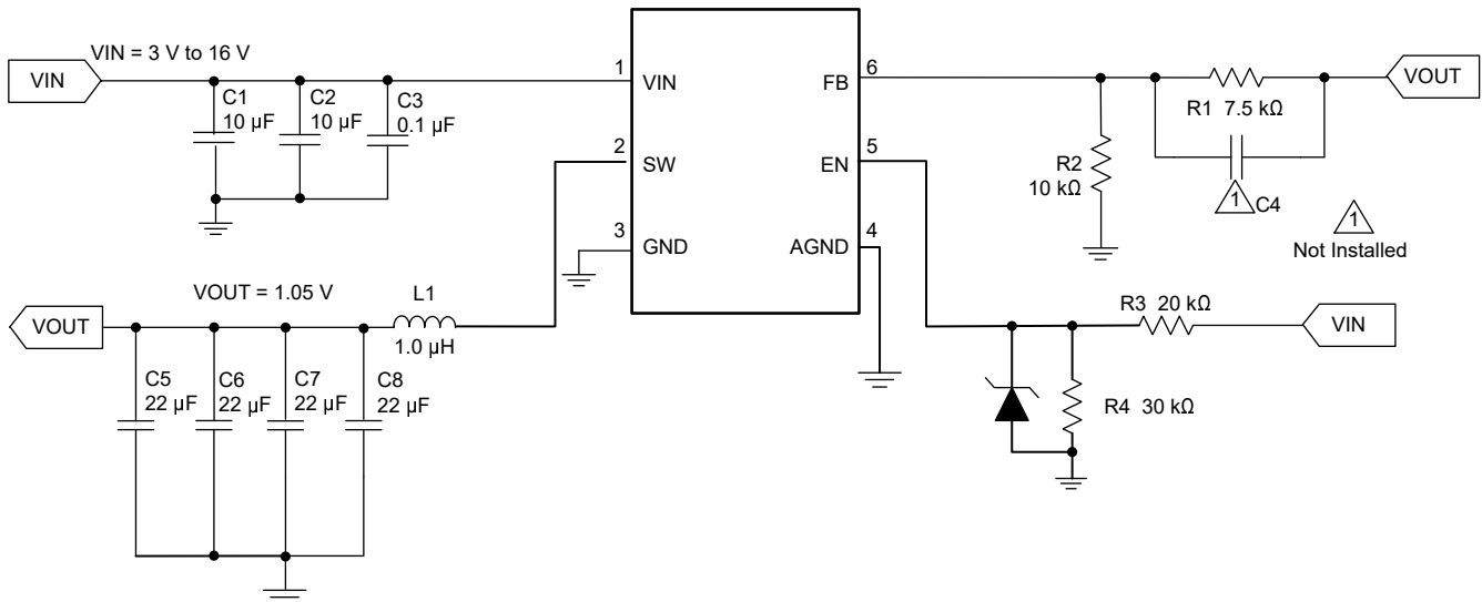
图 8-1. 原理图
