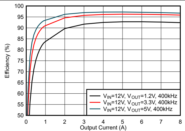
图 6-18. 效率, 模式 = FCCM, f_{SW} = 400kHz
