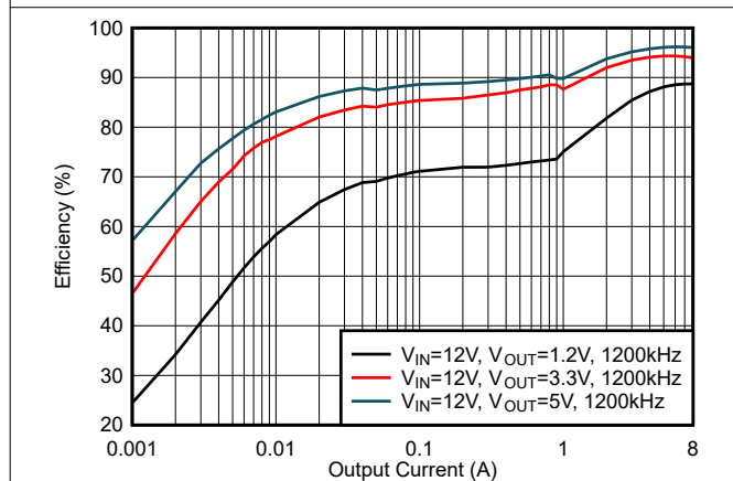
图 6-21. 效率, 模式 = DCM, f_{SW} = 1200kHz
