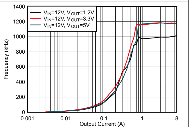
图 6-36. f_{SW} 负载调节, 模式 = DCM, f_{SW} = 1200kHz
