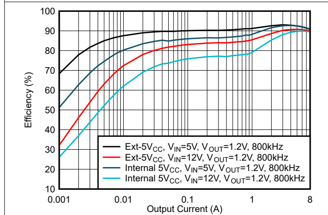
图 6-23. 效率, 外部 VCC 与内部 VCC, 模式 = DCM, f_{SW} = 800kHz
