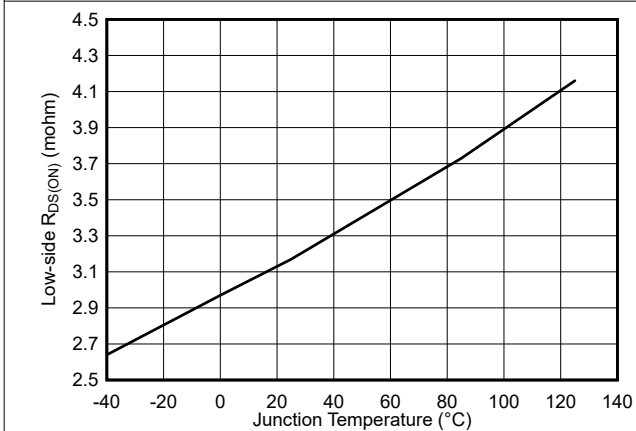
图 6-5. 低侧 R_{DS(on)} 与温度间的关系
