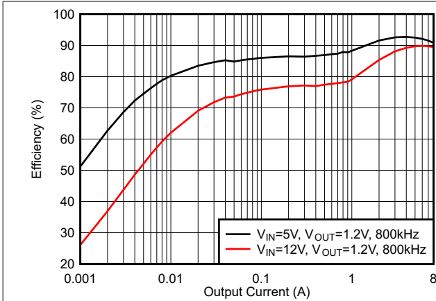
图 6-13. 效率, 模式 = DCM, f_{SW} = 800kHz
