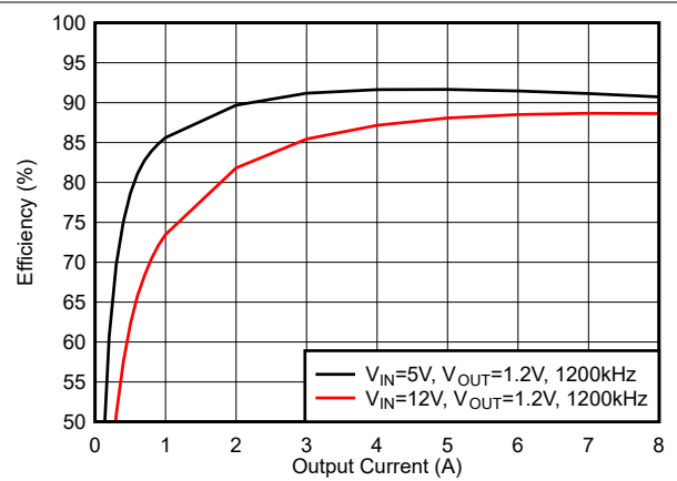
图 6-16. 效率, 模式 = FCCM, f_{SW} = 1200kHz
