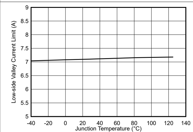
图 6-10. TPS568231 电流限制 (ILIM-1) 与温度间的关系
