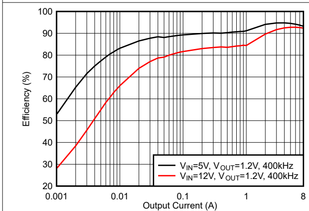
图 6-11. 效率, 模式 = DCM, f_{sw} = 400kHz
