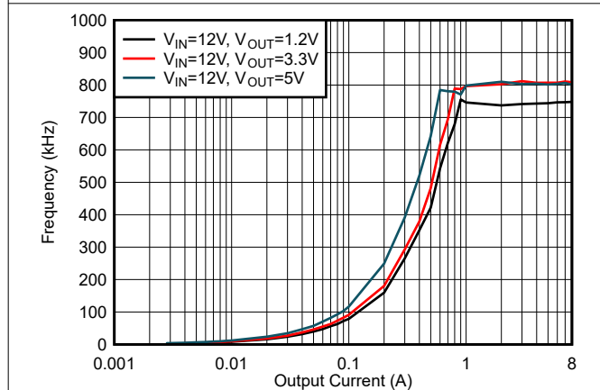
图 6-35. f_{SW} 负载调节, 模式 = DCM, f_{SW} = 800kHz
