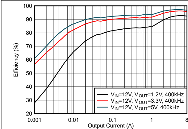
图 6-17. 效率, 模式 = DCM, f_{SW} = 400kHz
