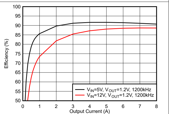
图 6-22. 效率, 模式 = FCCM, f_{SW} = 1200kHz
