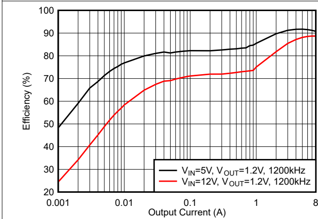
图 6-15. 效率, 模式 = DCM, f_{SW} = 1200kHz
