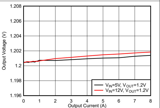
图 6-24. 负载调节, f_{SW} = 800kHz
