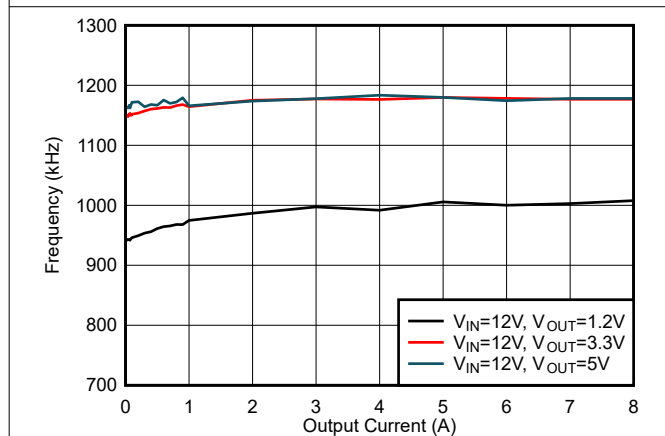
图 6-33. f_{SW} 负载调节, 模式 = FCCM, f_{SW} = 1200kHz
