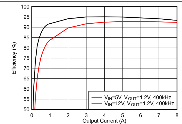
图 6-12. 效率, 模式 = FCCM, f_{sw} = 400kHz
