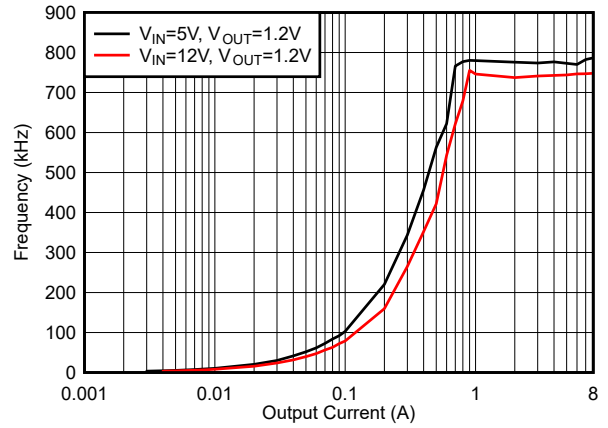
图 6-26. f_{SW} 负载调节, 模式 = DCM, f_{SW} = 800kHz
