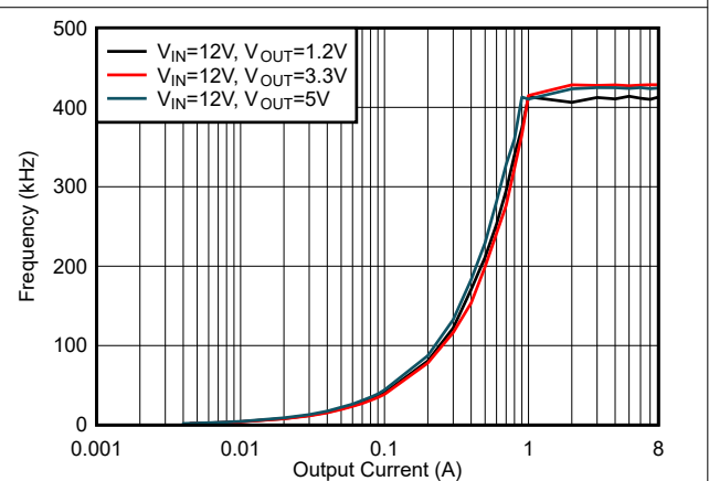
图 6-34. f_{SW} 负载调节, 模式 = DCM, f_{SW} = 400kHz
