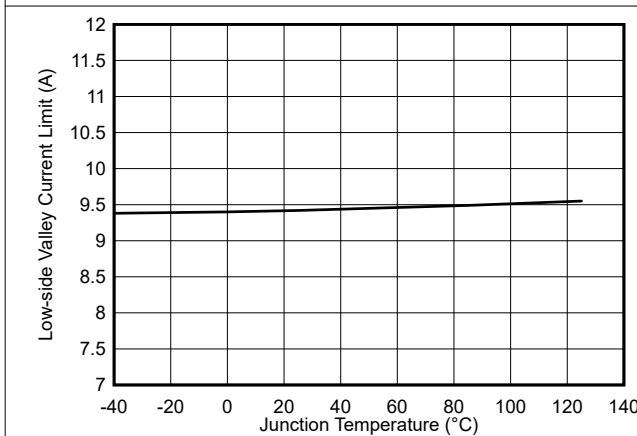
图 6-9. TPS568231 电流限制 (ILIM) 与温度间的关系
