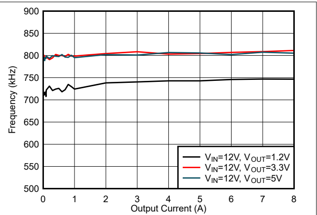
图 6-32. f_{SW} 负载调节, 模式 = FCCM, f_{SW} = 800kHz
