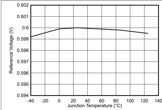
图 6-3. 基准电压与温度间的关系
