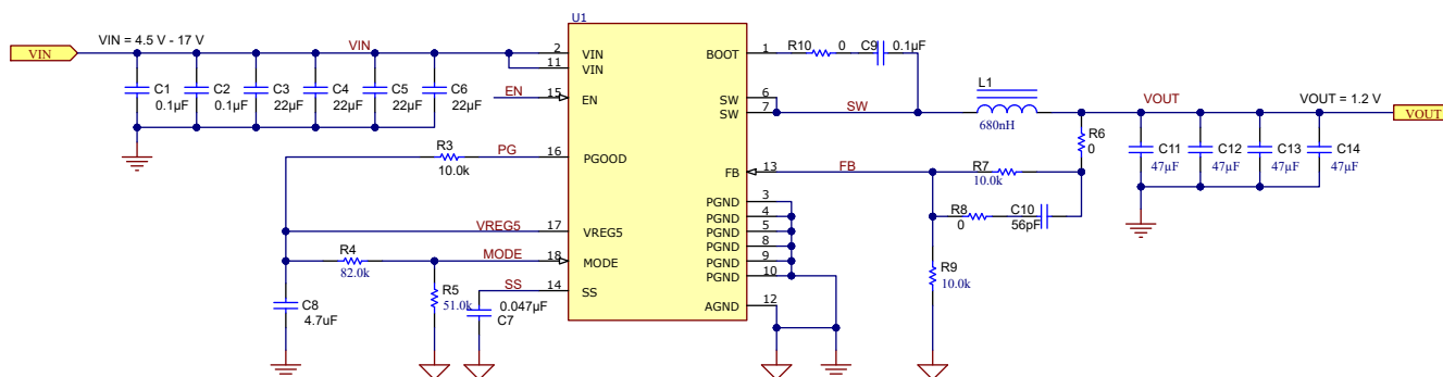
图 8-1. 应用原理图
