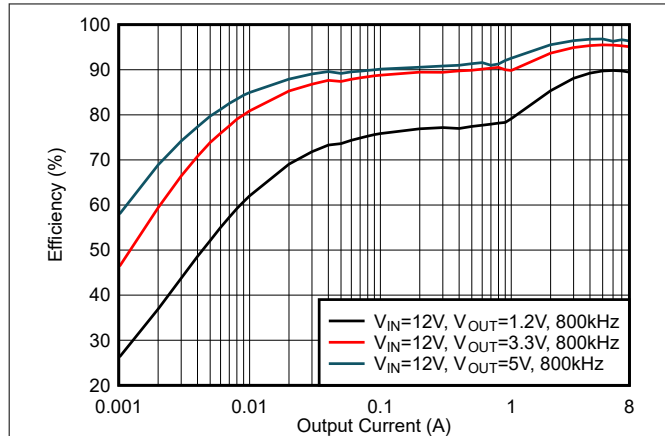
图 6-19. 效率, 模式 = DCM, f_{SW} = 800kHz
