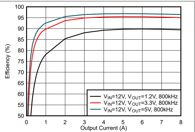
图 6-20. 效率, 模式 = FCCM, f_{SW} = 800kHz
