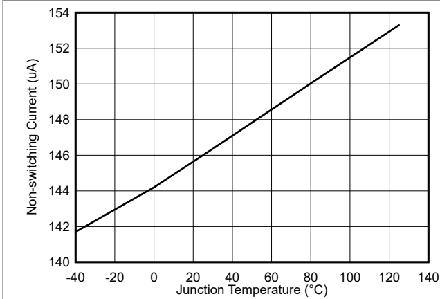
图 6-1. 静态电流与温度间的关系
