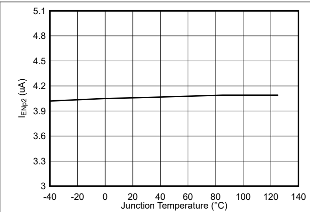
图 6-8. 使能上拉电流, V_{EN} = 1.3V
