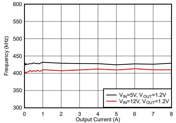
图 6-28. f_{SW} 负载调节, 模式 = FCCM, f_{SW} = 400kHz
