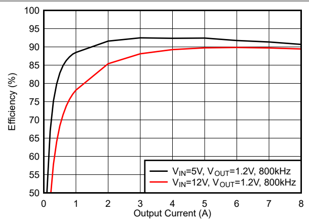
图 6-14. 效率, 模式 = FCCM, f_{SW} = 800kHz
