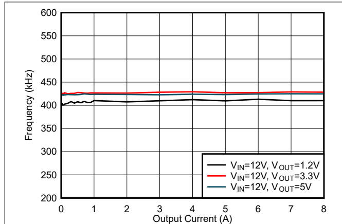
图 6-31. f_{SW} 负载调节, 模式 = FCCM, f_{SW} = 400kHz
