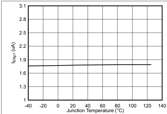
图 6-7. 使能上拉电流, V_{EN} = 1V
