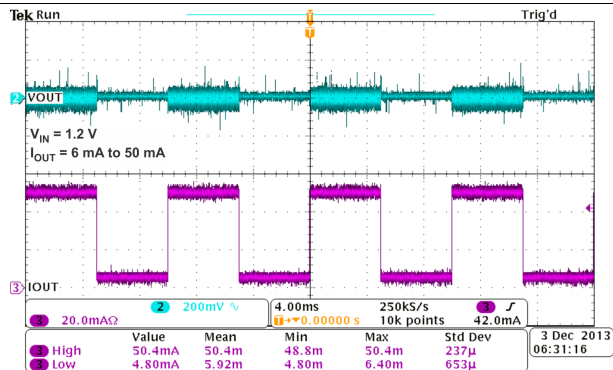
图 11. Load Transient Response
