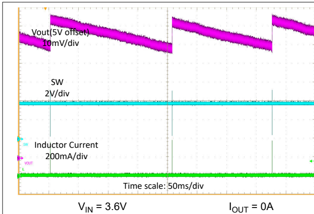
图 8-13. 开路负载时的开关波形
