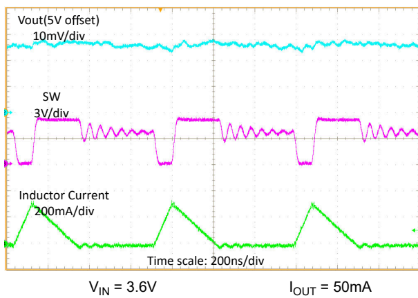
图 8-15. 中等负载条件下的开关波形
