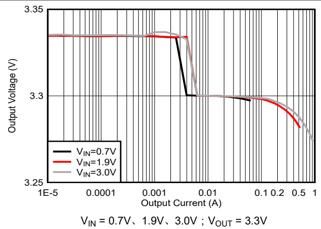
图 6-4. 正常模式下的 3.3V VOUT 负载调整率
