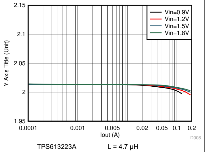
图 6-10. Load Regulation
