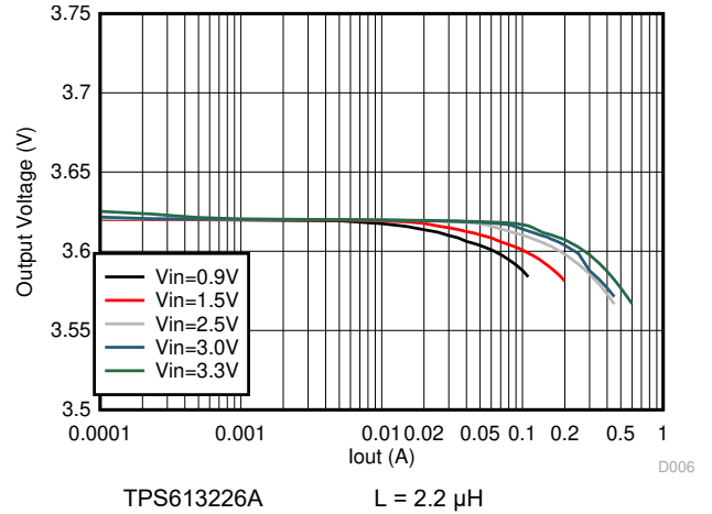
图 6-8. Load Regulation
