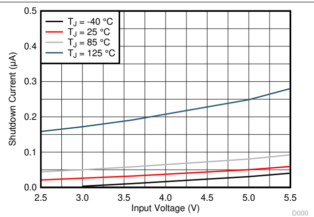
图 6-4. Shutdown Current
