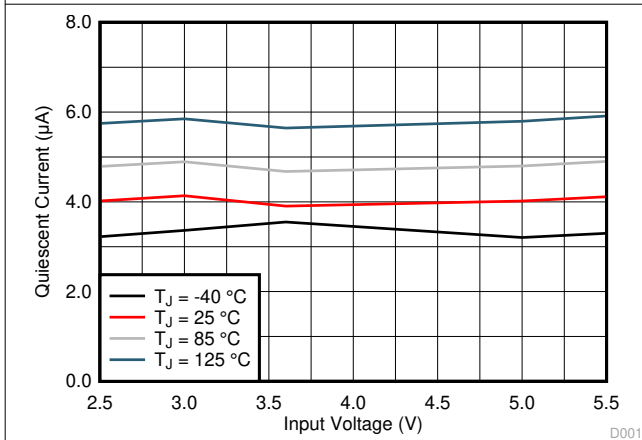
图 6-3. Quiescent Current
