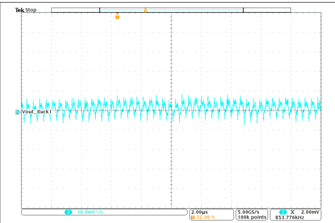
图 10-45. Output Voltage Ripple
