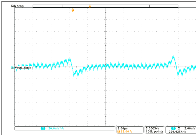
图 10-44. Ouput Voltage Ripple
