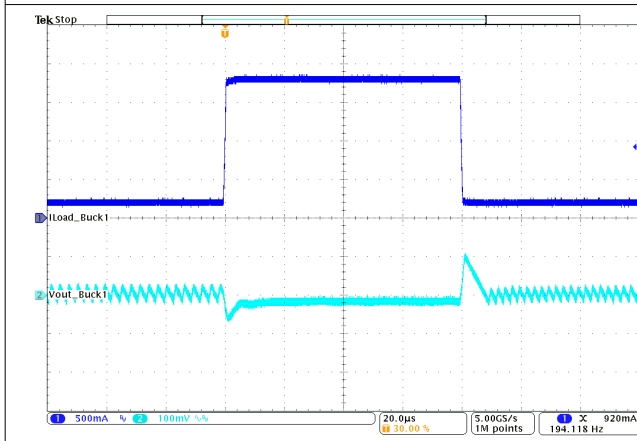
图 10-28. Load Transient Response
