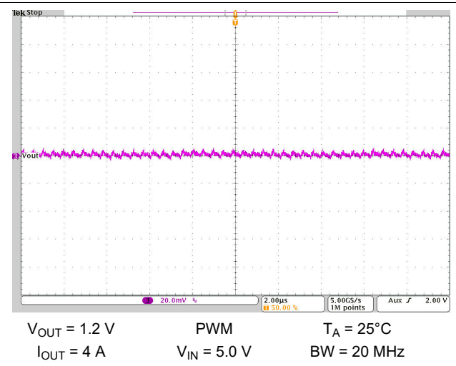
图 10-47. Output Voltage Ripple
