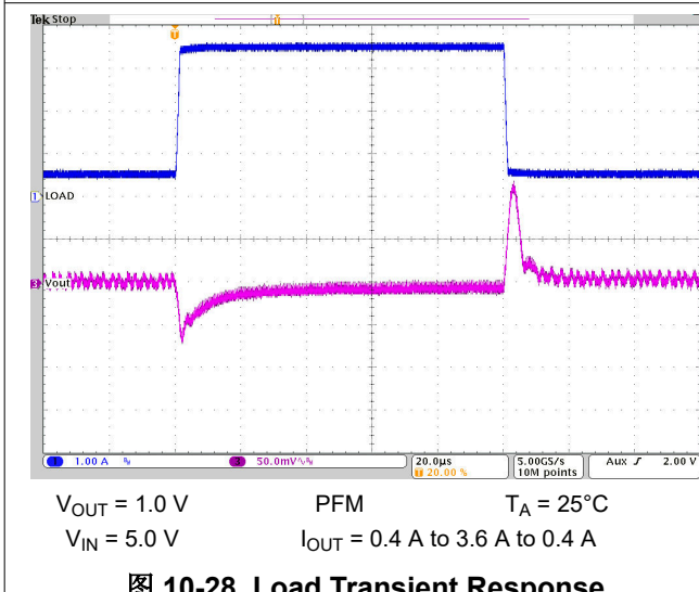
图 10-28. Load Transient Response
