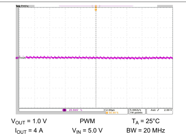
图 10-49. Output Voltage Ripple
