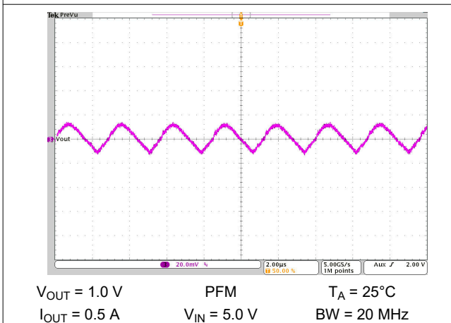
图 10-48. Output Voltage Ripple
