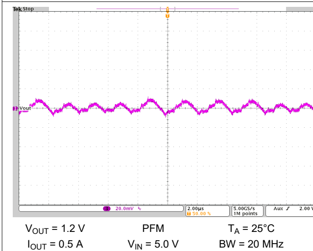
图 10-46. Output Voltage Ripple
