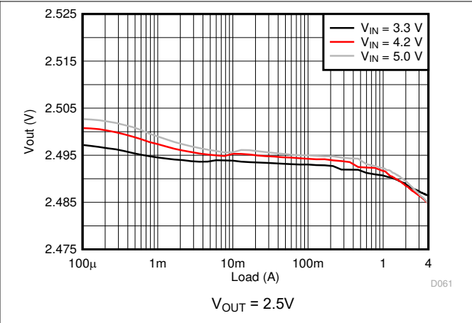
图 8-16. Load Regulation
