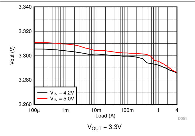
图 8-20. Load Regulation
