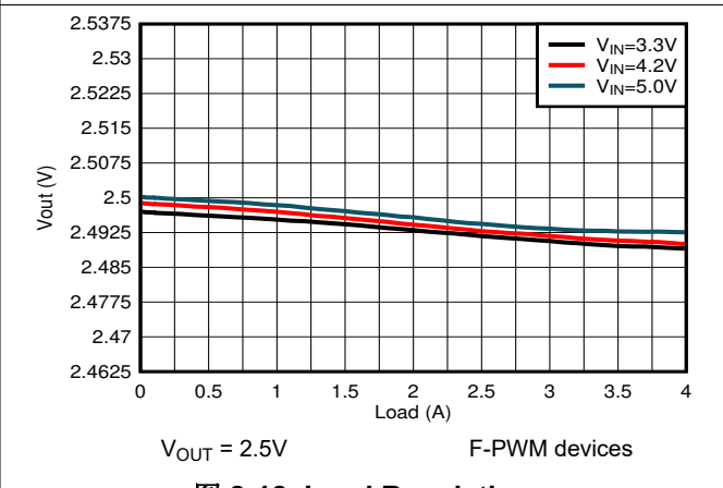
图 8-18. Load Regulation
