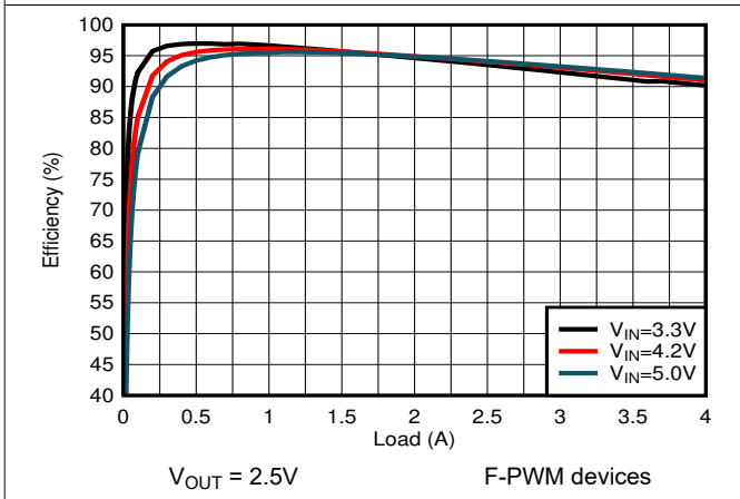
图 8-17. PWM Efficiency
