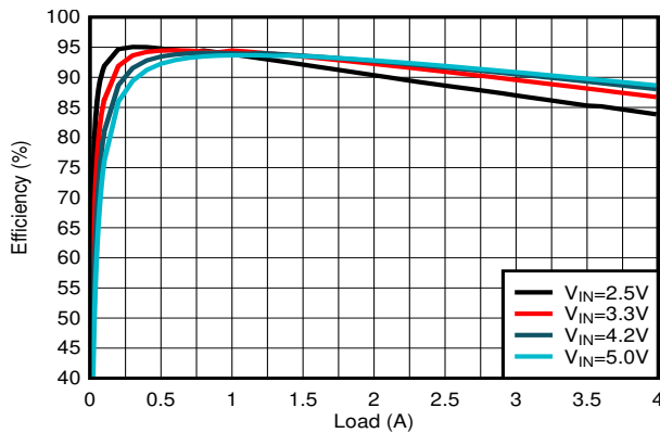
图 8-11. Efficiency
