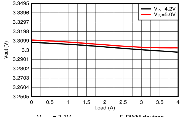
图 8-22. Load Regulation
