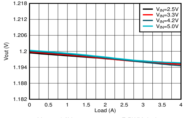
图 8-10. Load Regulation
