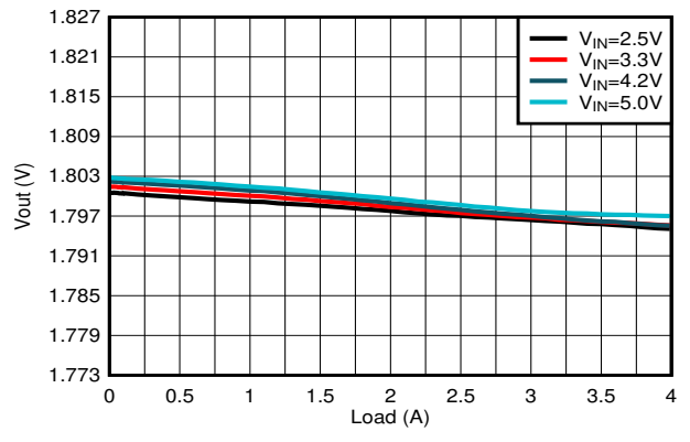
图 8-14. Load Regulation
