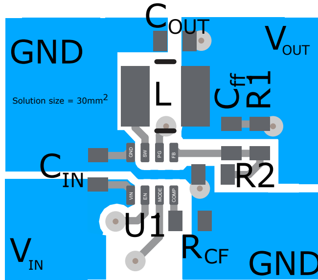
图 9-60. Example Layout
