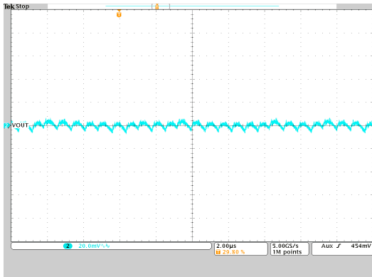
图 9-44. Output Voltage Ripple
