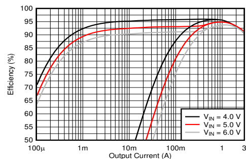
效率与 I_{OUT} 间的关系， V_{OUT} = 3.3\text{V}
