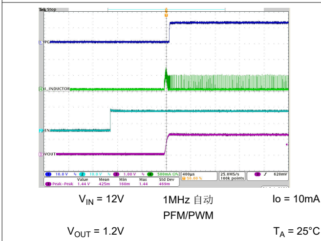
图 7-41. 启动时序
