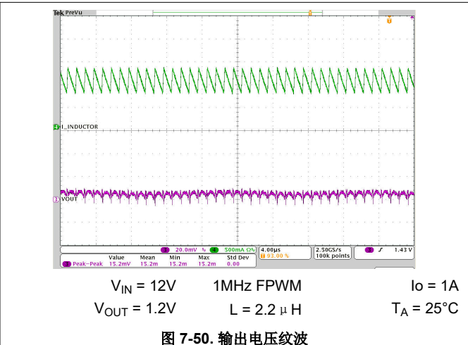
图 7-50. 输出电压纹波
