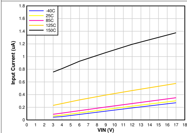
图 5-3. 典型关断电流
