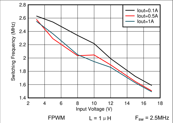
图 7-38. 开关频率与输入电压间的关系 V OUT = 1.2V
