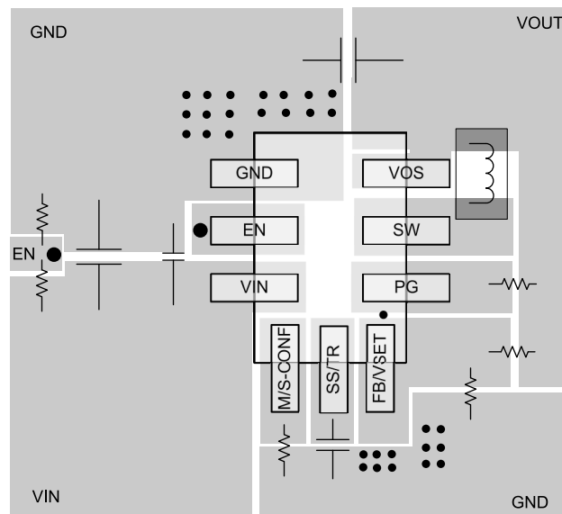
图 7-85. 布局
