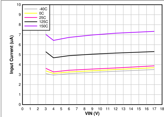
图 5-1. 典型静态电流与 V_{IN} 间的关系
