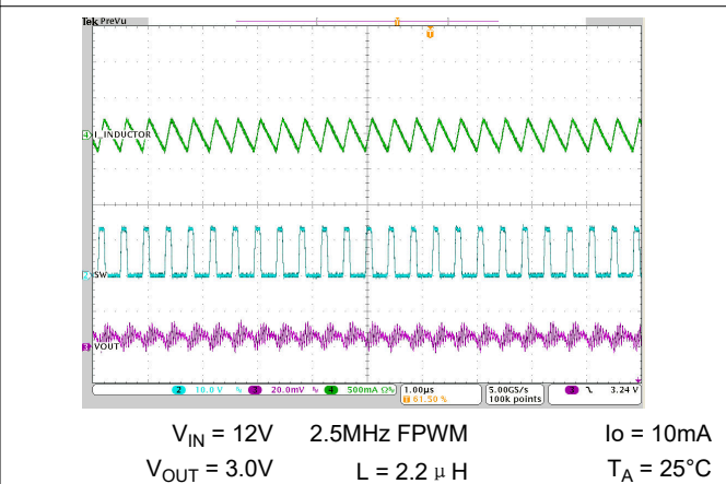
图 7-54. 典型操作
