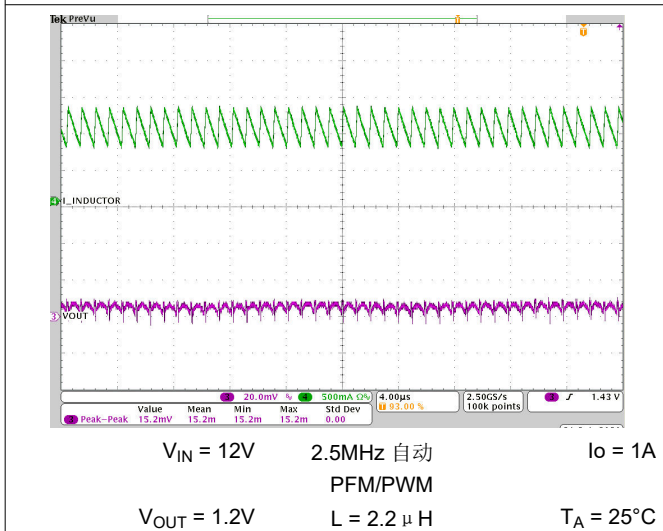
图 7-51. 输出电压纹波
