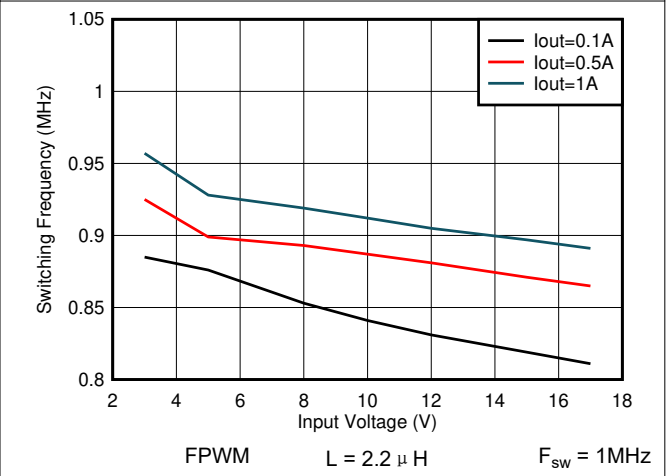
图 7-36. 开关频率与输入电压间的关系 V OUT = 1.2V
