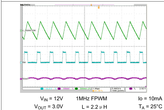
图 7-53. 典型操作
