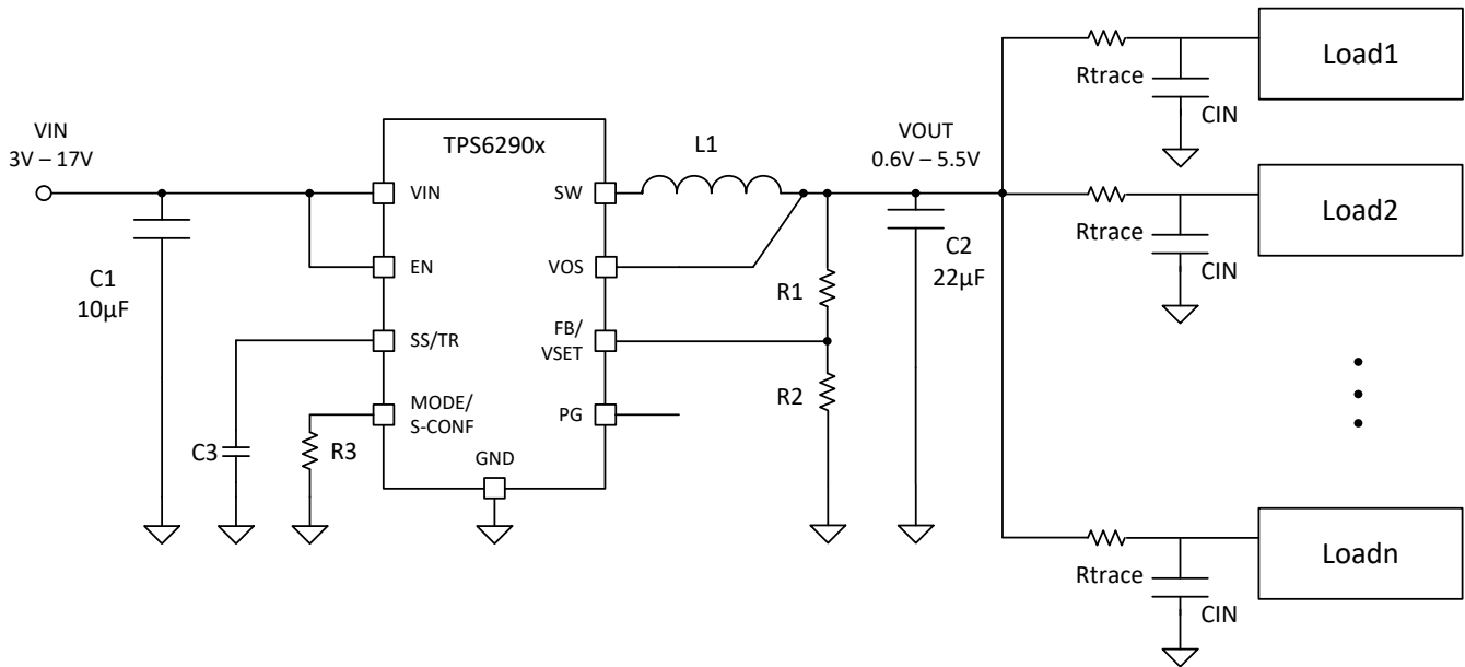
图 7-82. 多个负载
