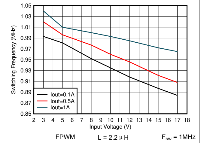
图 7-32. 开关频率与输入电压间的关系 V OUT = 1.8V
