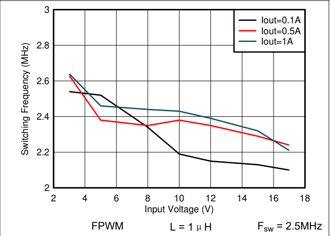
图 7-34. 开关频率与输入电压间的关系 V OUT = 1.8V
