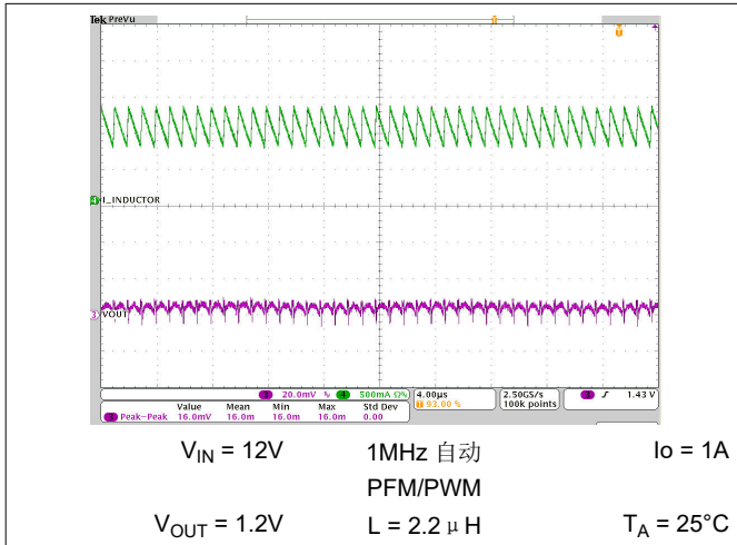
图 7-49. 输出电压纹波
