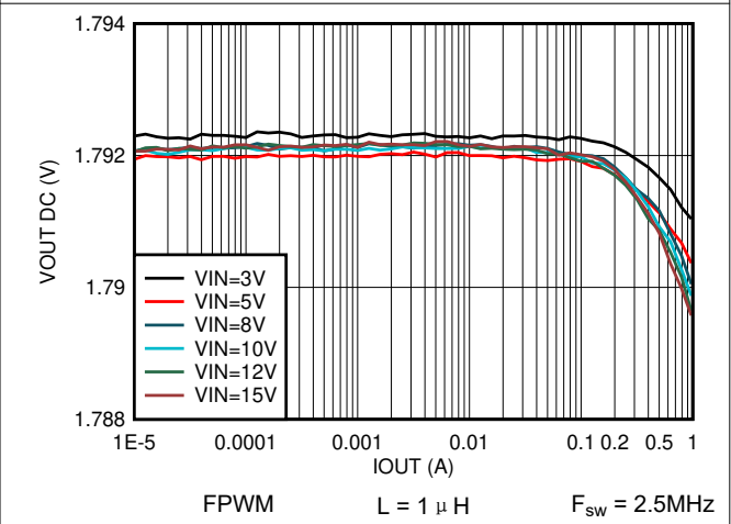
图 7-40. 输出电压与输出电流间的关系 V OUT = 1.8V
