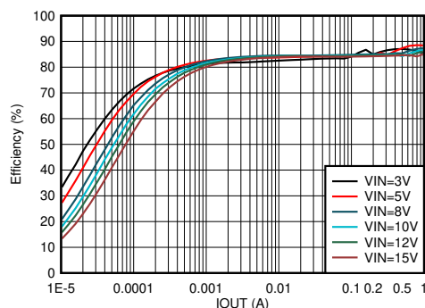
效率与输出电流间的关系 (1.2V O , 2.5MHz-1 μH, 自动 PFM/PWM)
