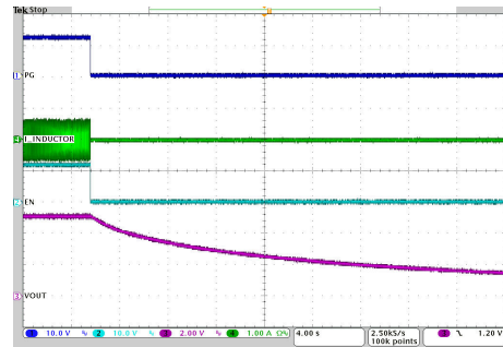
图 7-64. 输出放电功能 - 禁用
