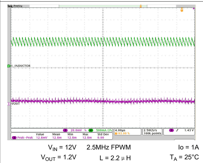
图 7-52. 输出电压纹波
