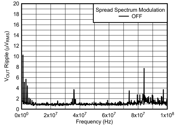
12V 至 1.2V, 2A 1 \mu H, 1MHz 第 1 和第 2 个 L-C BW = 10kHz 图 5-4. 第 2 个 L-C 滤波器之后的 V_{OUT} 纹波 FFT
