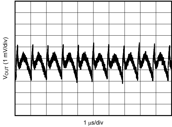
12V 至 1.2V, 2A 1 \mu H, 1MHz 仅第 1 个 L-C 图 5-1. 第 1 个 L-C 滤波器之后的 V_{OUT} 纹波
