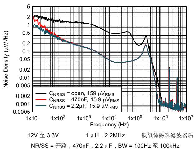
图 5-18. 输出噪声密度与频率间的关系
