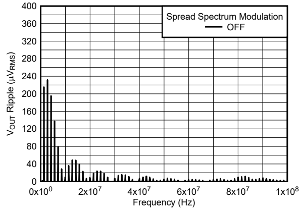
12V 至 1.8V, 2A 1 \mu H, 1.4MHz 仅第 1 个 L-C BW = 10kHz 图 5-6. 第 1 个 L-C 滤波器之后的 V_{OUT} 纹波 FFT
