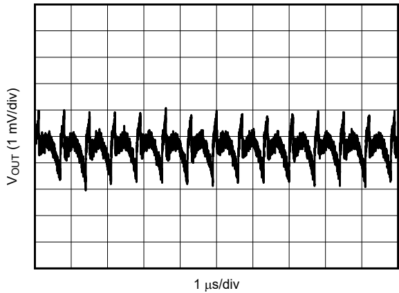
12V 至 1.8V, 2A 1 \mu H, 1.4MHz 仅第 1 个 L-C 图 5-5. 第 1 个 L-C 滤波器之后的 V_{OUT} 纹波
