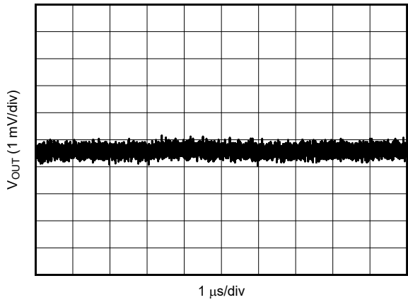
12V 至 1.2V, 2A 1 \mu H, 1MHz 第 1 和第 2 个 L-C 图 5-3. 第 2 个 L-C 滤波器之后的 V_{OUT} 纹波
