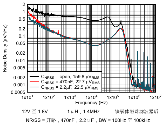
图 5-16. 输出噪声密度与频率间的关系
