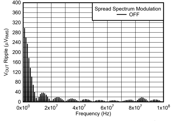
12V 至 1.2V, 2A 1 \mu H, 2MHz 仅第 1 个 L-C BW = 10kHz 图 5-2. 第 1 个 L-C 滤波器之后的 V_{OUT} 纹波 FFT
