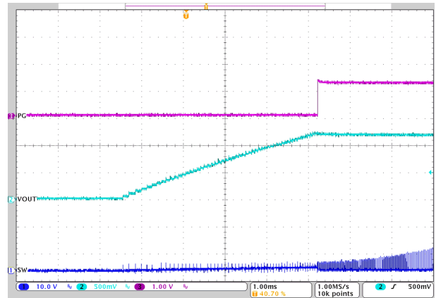
NR/SS = 470nF 12V 至 1.2V 1 \mu H, 1MHz 1A 负载
