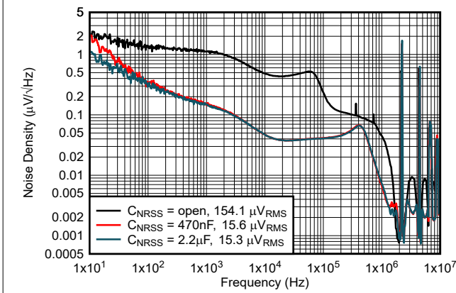
图 5-15. 输出噪声密度与频率间的关系
