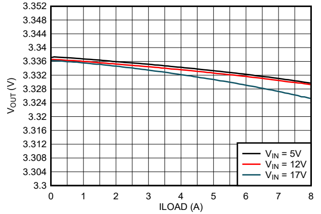
3.3Vout 1 \mu H, 2.2MHz 仅第 1 个 L-C
