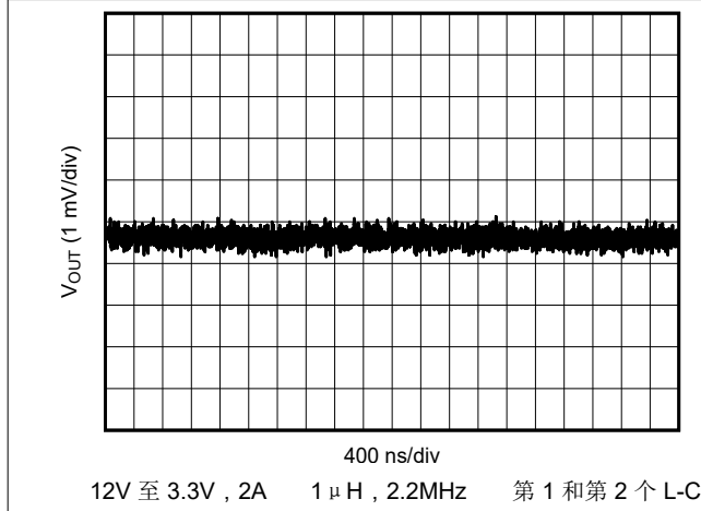
图 5-11. 第 2 个 L-C 滤波器之后的 V_{OUT} 纹波
