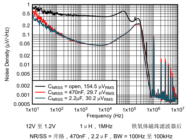
图 5-14. 输出噪声密度与频率间的关系
