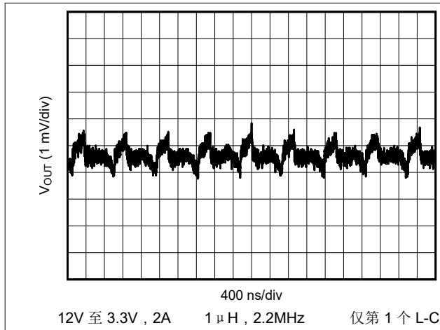
图 5-9. 第 1 个 L-C 滤波器之后的 V_{OUT} 纹波
