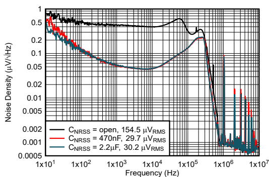
输出噪声与频率间的关系
