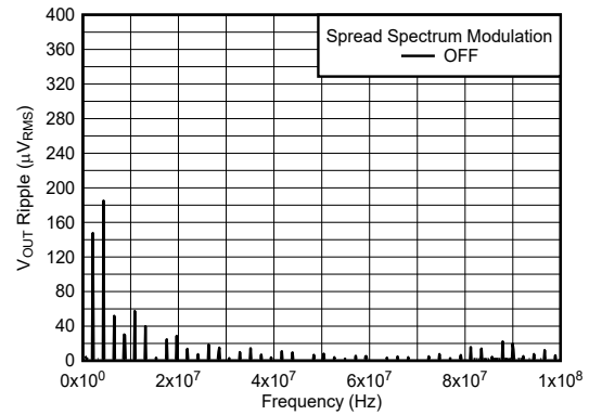
12V 至 3.3V, 2A 1 \mu H, 2.2MHz 仅第 1 个 L-C BW = 10kHz 图 5-10. 第 1 个 L-C 滤波器之后的 V_{OUT} 纹波 FFT
