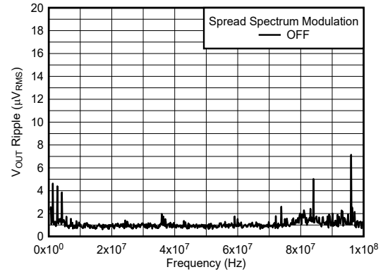
12V 至 1.8V, 2A 1 \mu H, 1.4MHz 第 1 和第 2 个 L-C BW = 10kHz 图 5-8. 第 2 个 L-C 滤波器之后的 V_{OUT} 纹波 FFT
