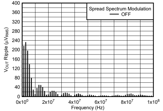
图 5-4. 第 2 个 L-C 滤波器之后的 V_{OUT} 纹波 FFT
