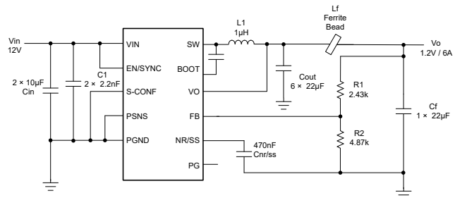
典型应用
