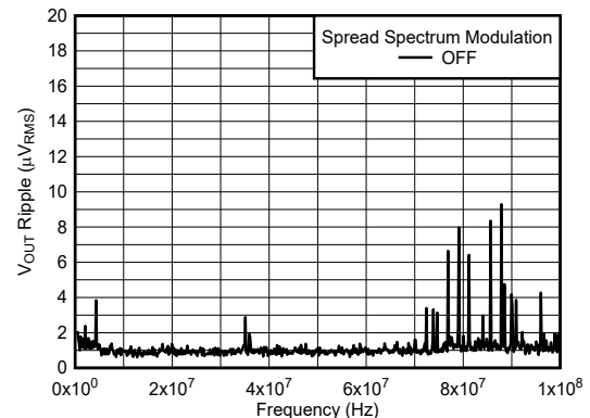
12V 至 3.3V, 2A 1 \mu H, 2.2MHz 第 1 和第 2 个 L-C BW = 10kHz 图 5-12. 第 2 个 L-C 滤波器之后的 V_{OUT} 纹波 FFT
