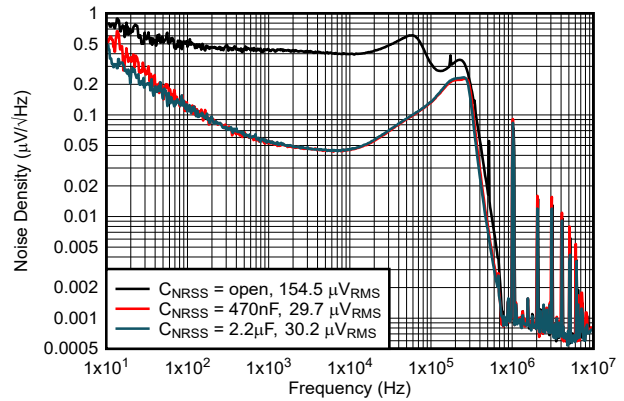
图 5-14. 输出噪声密度与频率间的关系
