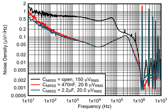
图 5-13. 输出噪声密度与频率间的关系
