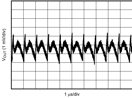
图 5-1. 第 1 个 L-C 滤波器之后的 V_{OUT} 纹波
