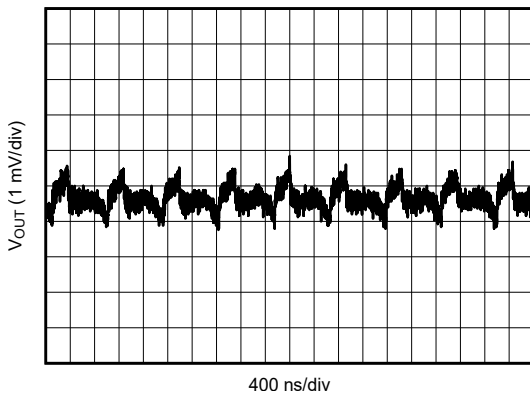
12V 至 3.3V, 2A 1 \mu H, 2.2MHz 仅第 1 个 L-C 图 5-9. 第 1 个 L-C 滤波器之后的 V_{OUT} 纹波
