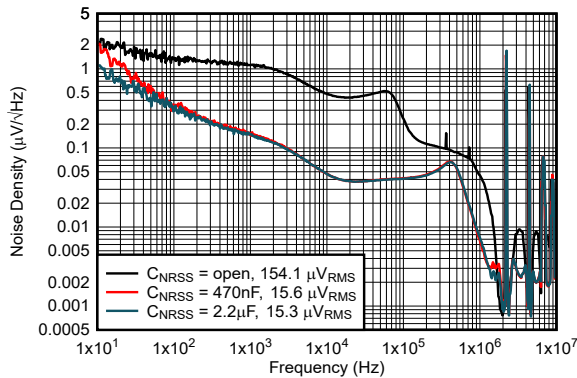
图 5-15. 输出噪声密度与频率间的关系
