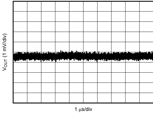
图 5-3. 第 2 个 L-C 滤波器之后的 V_{OUT} 纹波
