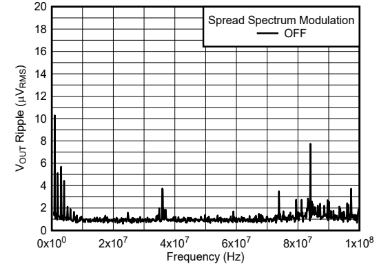
图 5-2. 第 1 个 L-C 滤波器之后的 V_{OUT} 纹波 FFT
