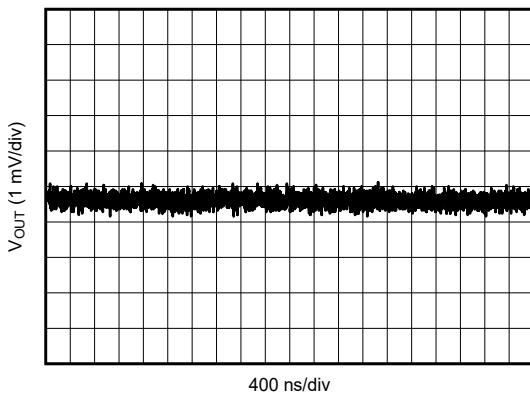
12V 至 3.3V, 2A 1 \mu H, 2.2MHz 第 1 和第 2 个 L-C 图 5-11. 第 2 个 L-C 滤波器之后的 V_{OUT} 纹波
