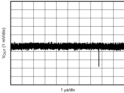
12V 至 1.8V, 2A 1 \mu H, 1.4MHz 第 1 和第 2 个 L-C 图 5-7. 第 2 个 L-C 滤波器之后的 V_{OUT} 纹波
