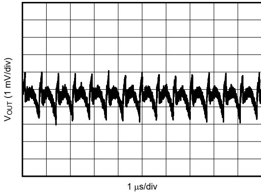
图 5-5. 第 1 个 L-C 滤波器之后的 V_{OUT} 纹波
