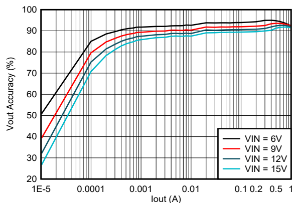
效率与输出电流间的关系 (频率为 1.0MHz 时 V_{OUT} = 3.3V , 自动 PFM/PWM)
